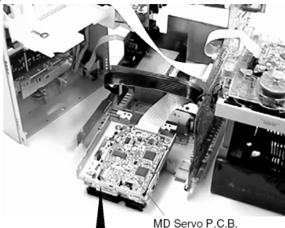
MD Servo P.C.B.
