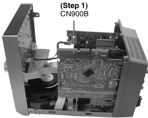
Step 1: Detach connector (CN900B).
