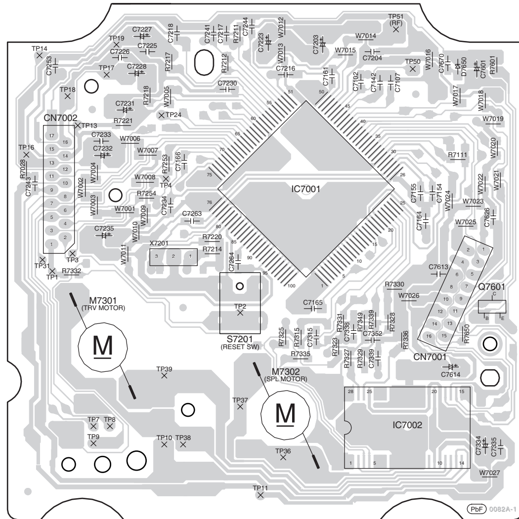
A CD SERVO P.C.B (REPV0082A)
