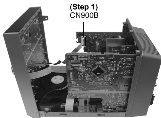
Step 1: Detach connector (CN900B).
