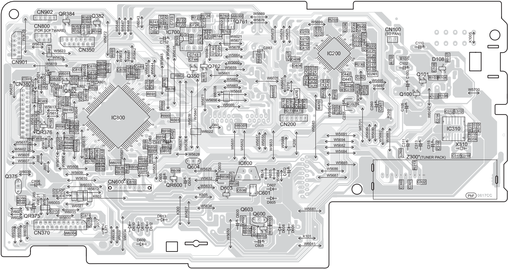
B MAIN P.C.B. (REPX0849HC)
