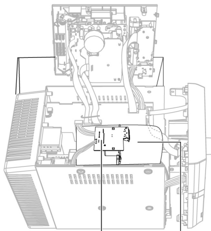
Power P.C.B. (Step 15)
