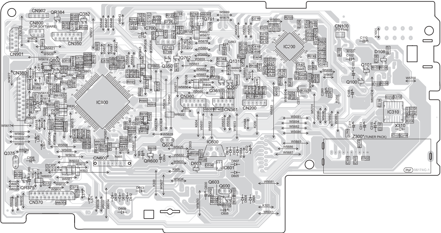
B MAIN P.C.B. (REPX0708A)
