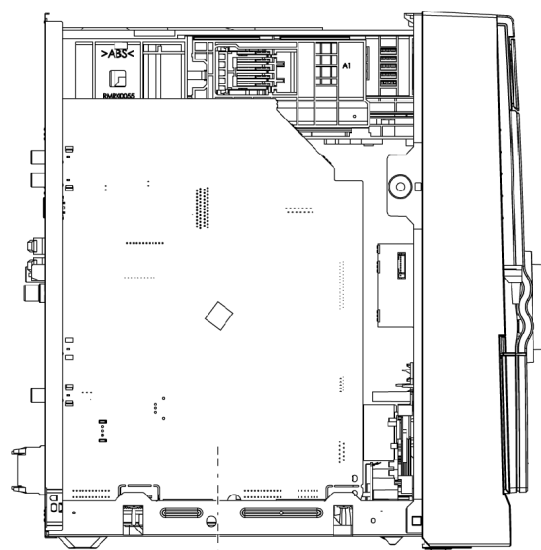
Main P.C.B.
