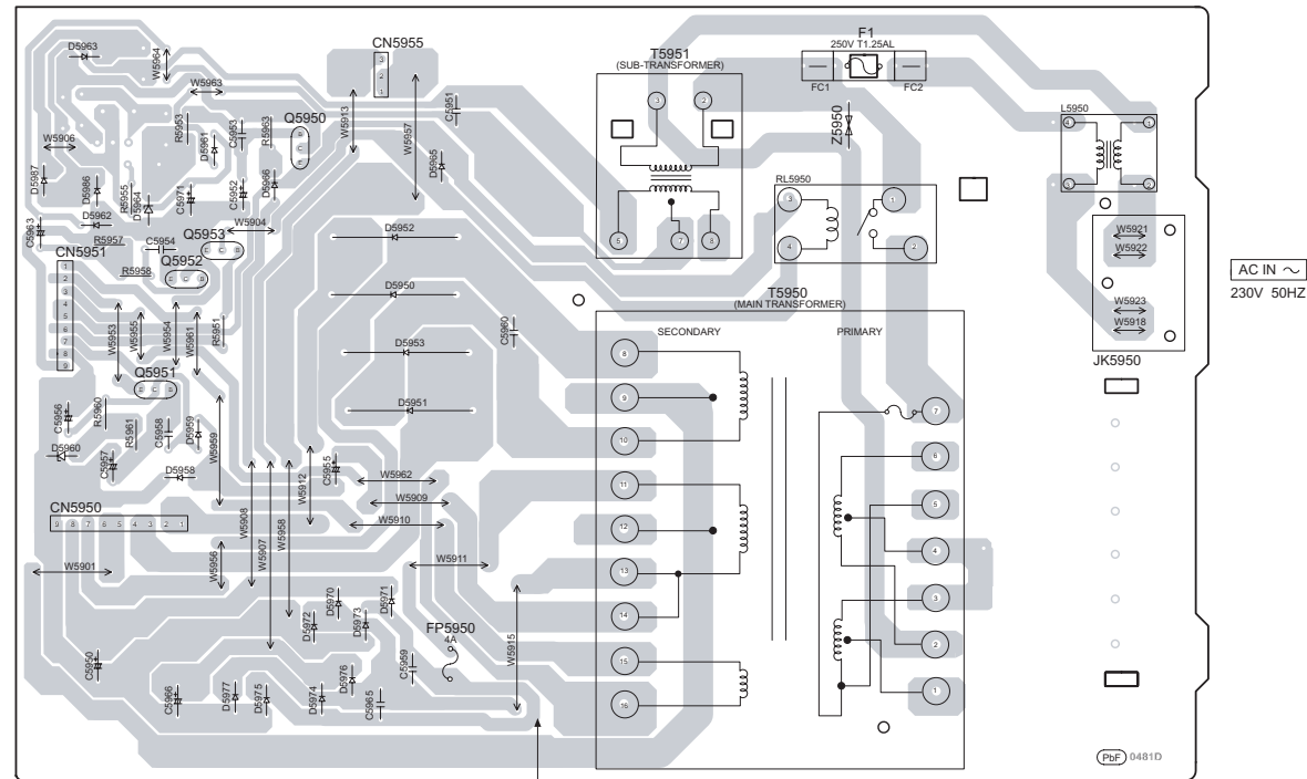
I SMPS P.C.B. (REPX0519E)
