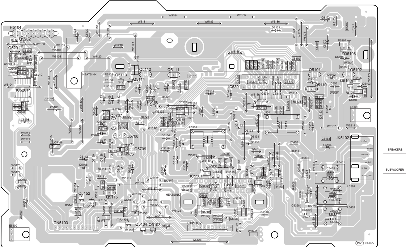
H D-AMP P.C.B. (REPV0138B)
