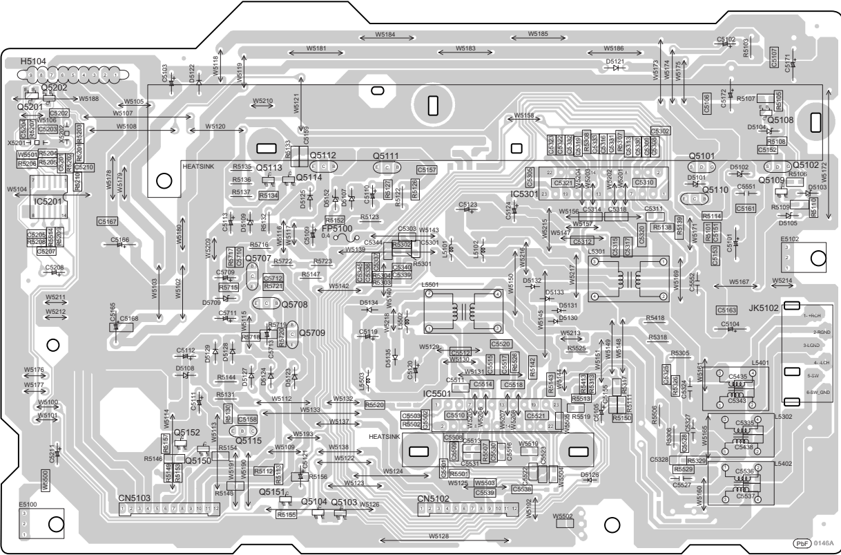
H D-AMP P.C.B. (REPV0138B)
