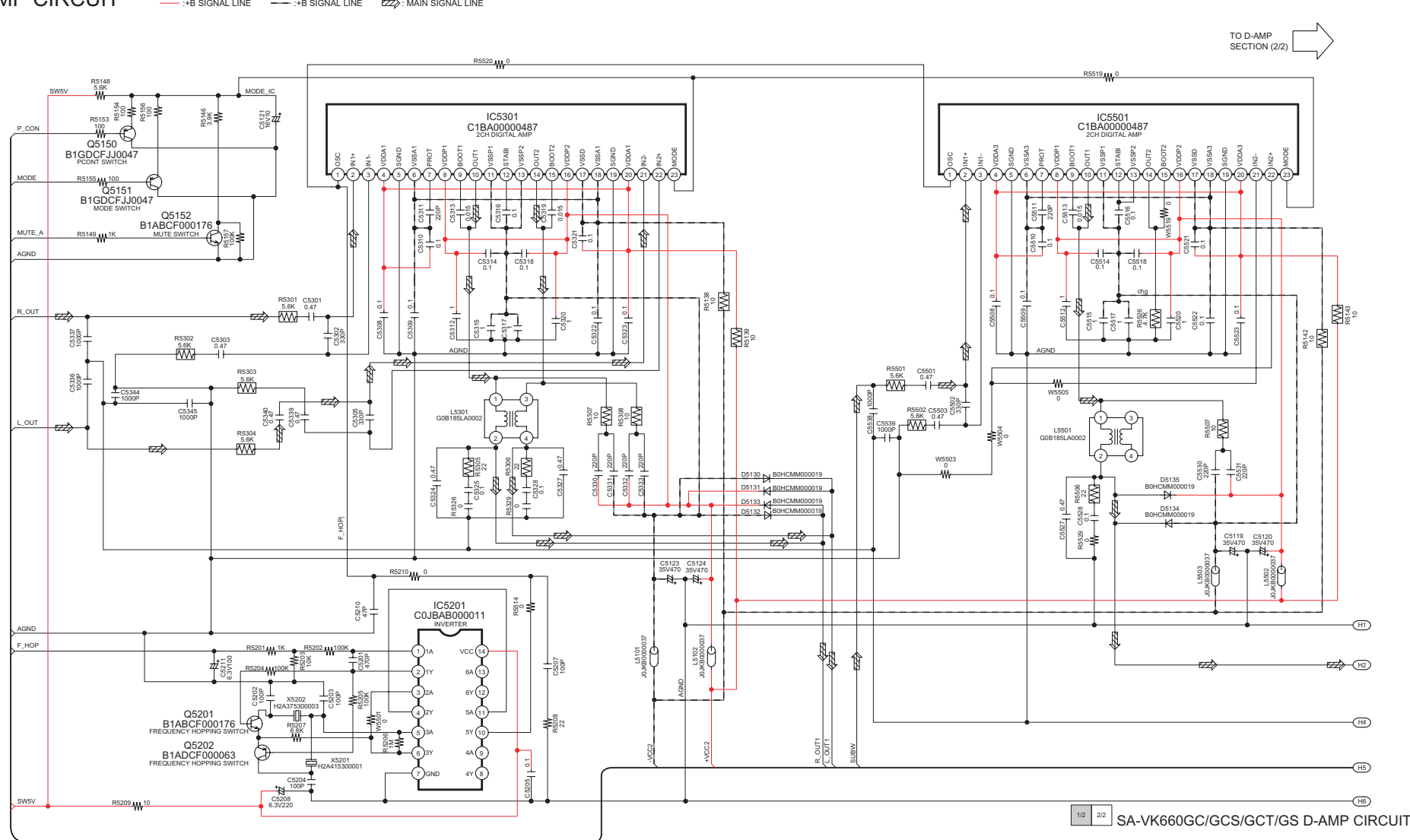
H D-AMP CIRCUIT
