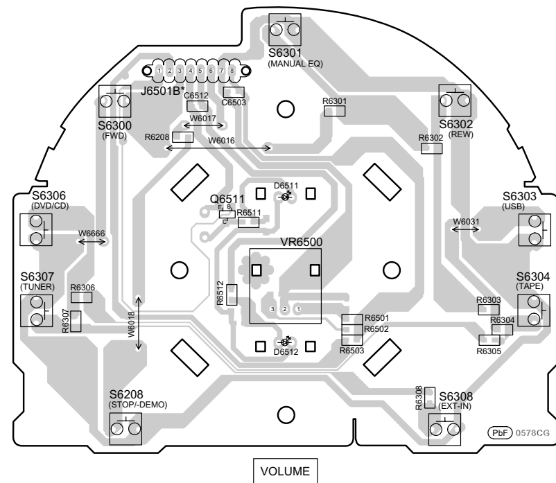
F VOLUME P.C.B. (REPX0737B)
