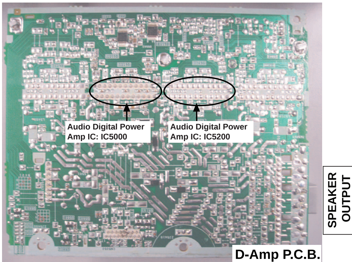
Figure 3 D-Amp P.C.B.
