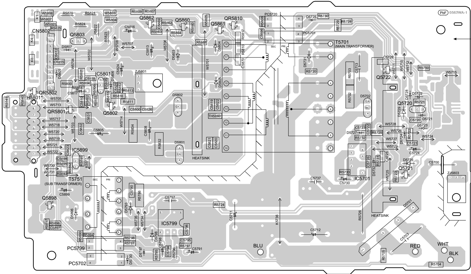
N SMPS P.C.B. (REPX0751H)
