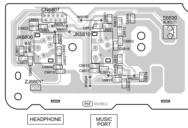
G MUSIC PORT P.C.B. (REPX0737B)
