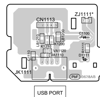
J USB P.C.B. (REPX0736H)
