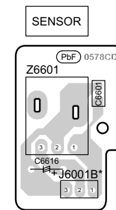
H REMOTE SENSOR P.C.B. (REPX0737B)
