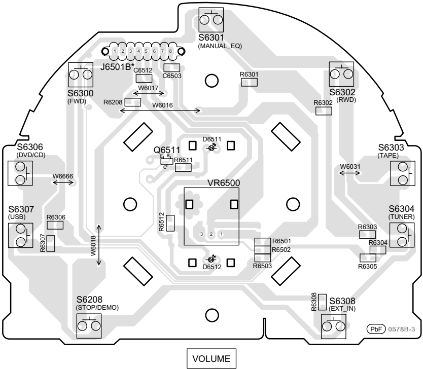
F TACT SWITCH P.C.B. (REPX0671C)
