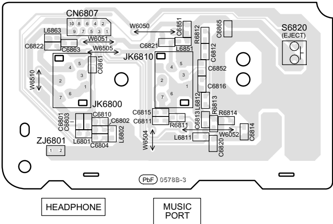
G MUSIC PORT P.C.B. (REPX0671C)
