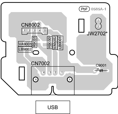
J USB P.C.B. (REPX0659C)
