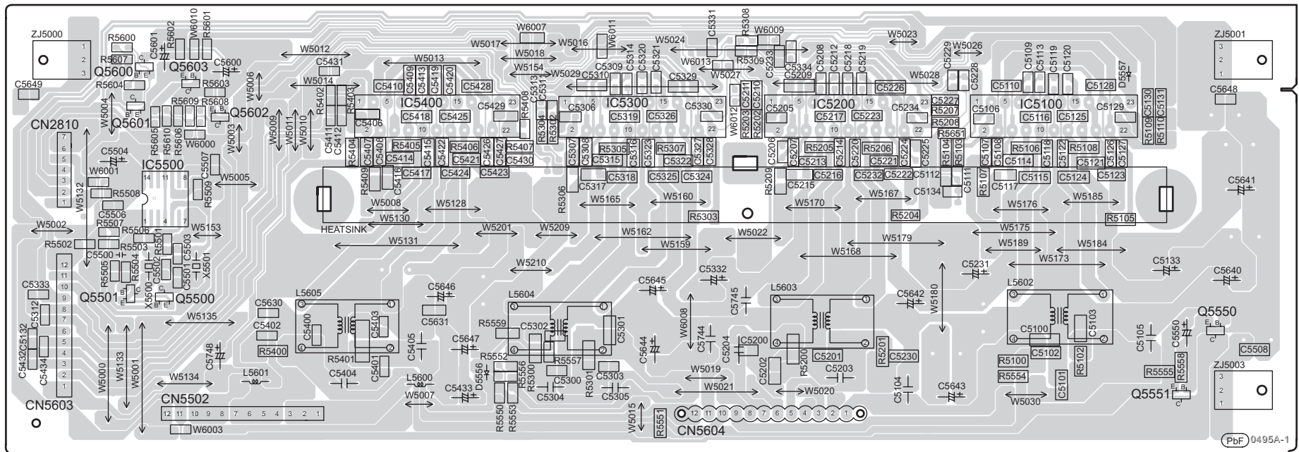
J D-AMP P.C.B. (REPV0144A)
