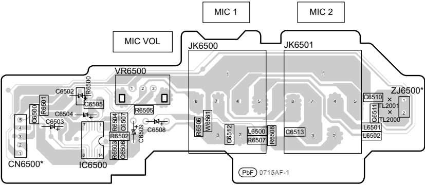
G USB P.C.B. (REPX0877BB)
