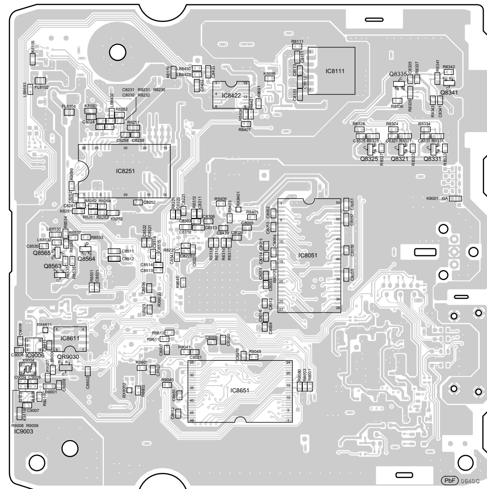
A DVD MODULE P.C.B. (RFKBX0885A...GC/GS) (RFKBX0885B...GA)
