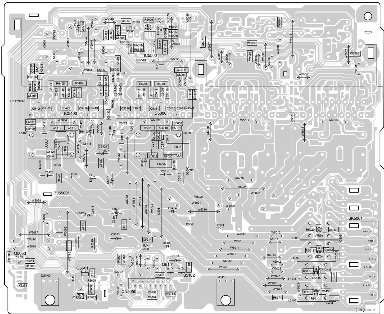
I D-AMP P.C.B. (REPX0821E)
