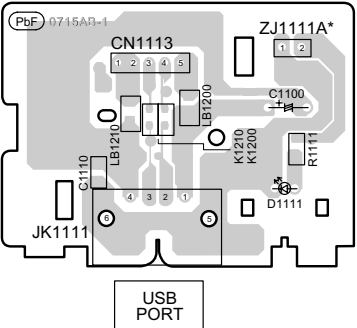
H REMOTE SENSOR P.C.B. (REPX0877BC)
