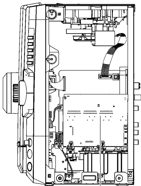
D-Amp P.C.B. (Step 2)
