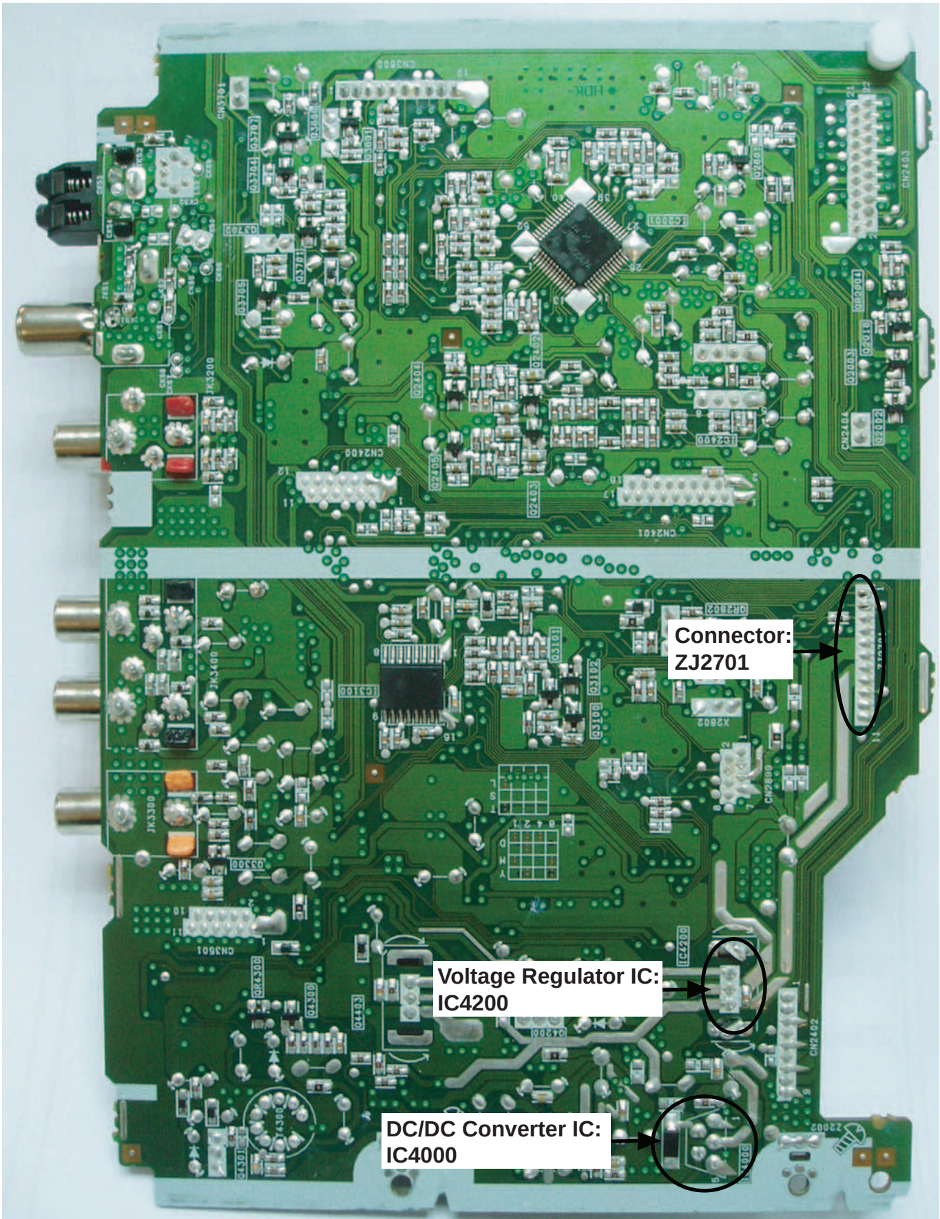
Fig. 2 Main P.C.B.
