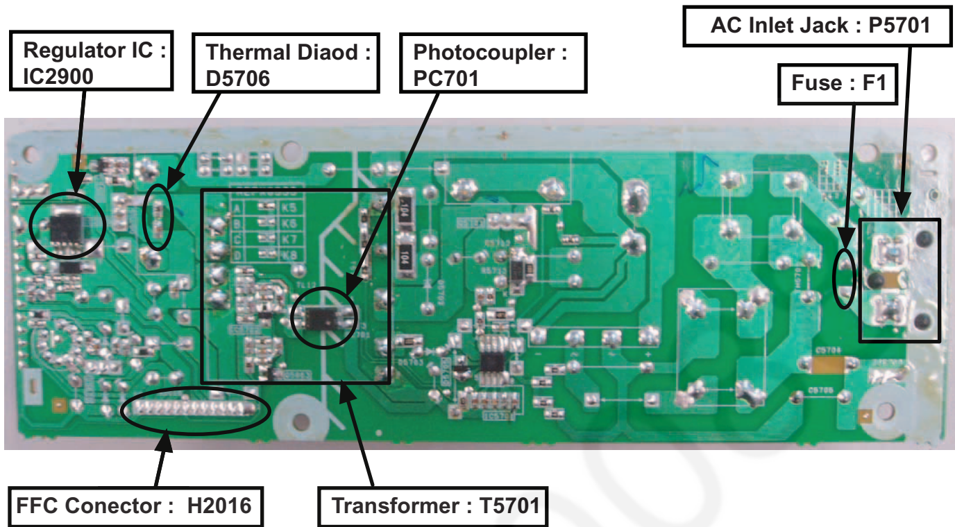
Fig. 1. SMPS P.C.B.
