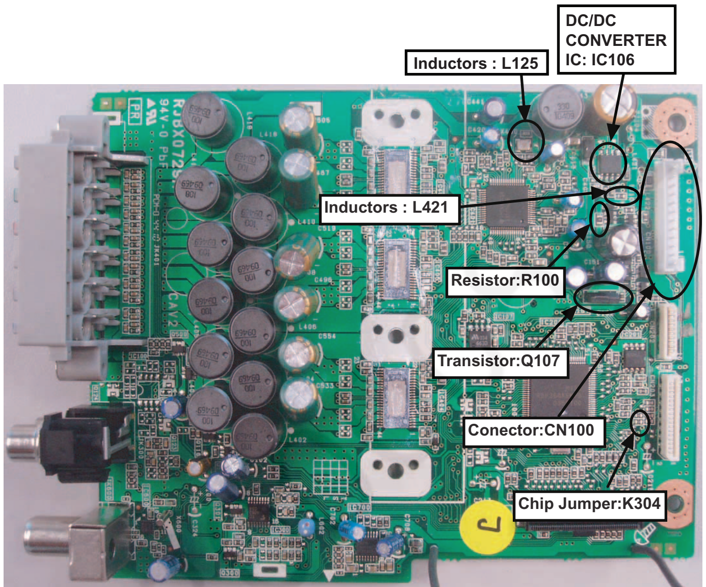
Fig. 2. Main P.C.B.
