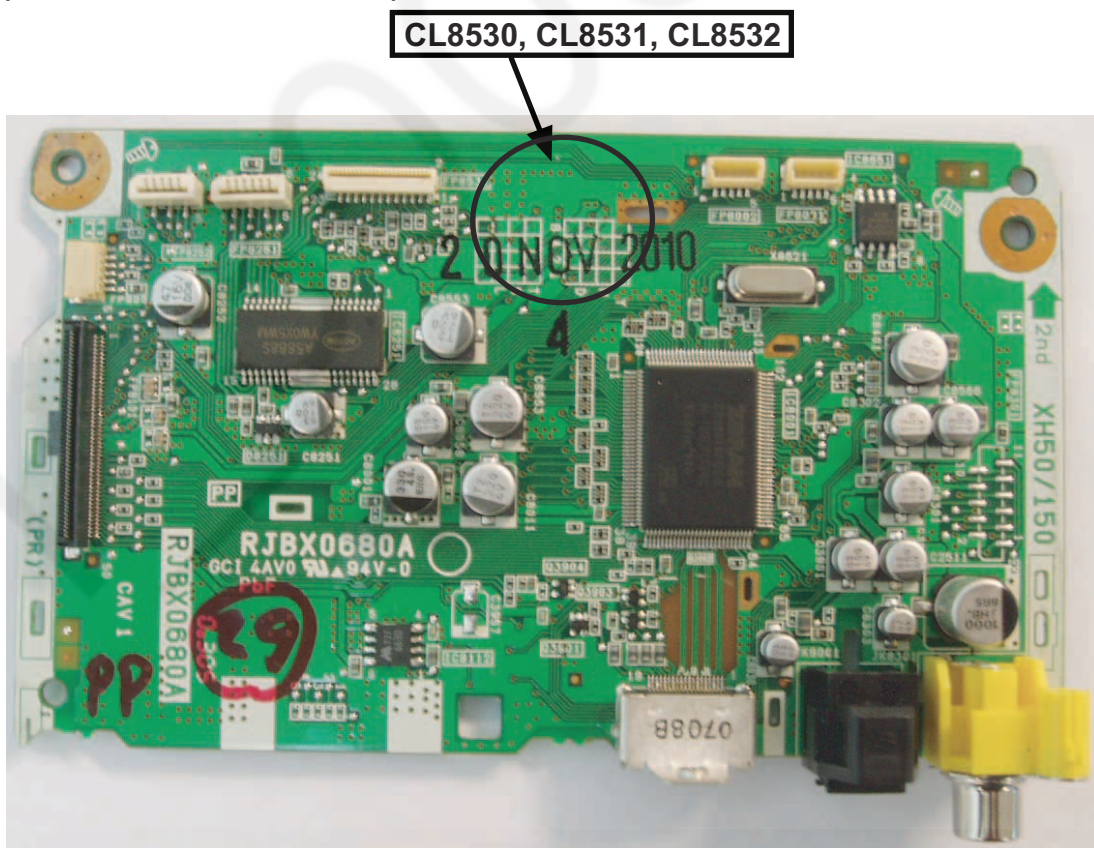
Fig. 3. Backend P.C.B.
