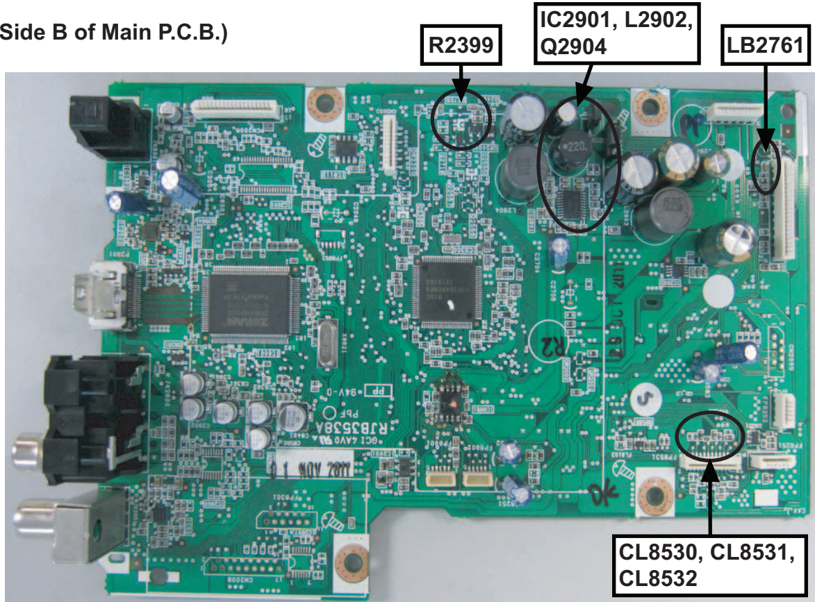
Fig. 2. Main P.C.B.
