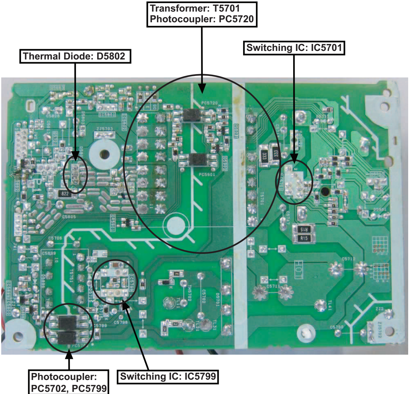
Fig. 1. SMPS P.C.B.
