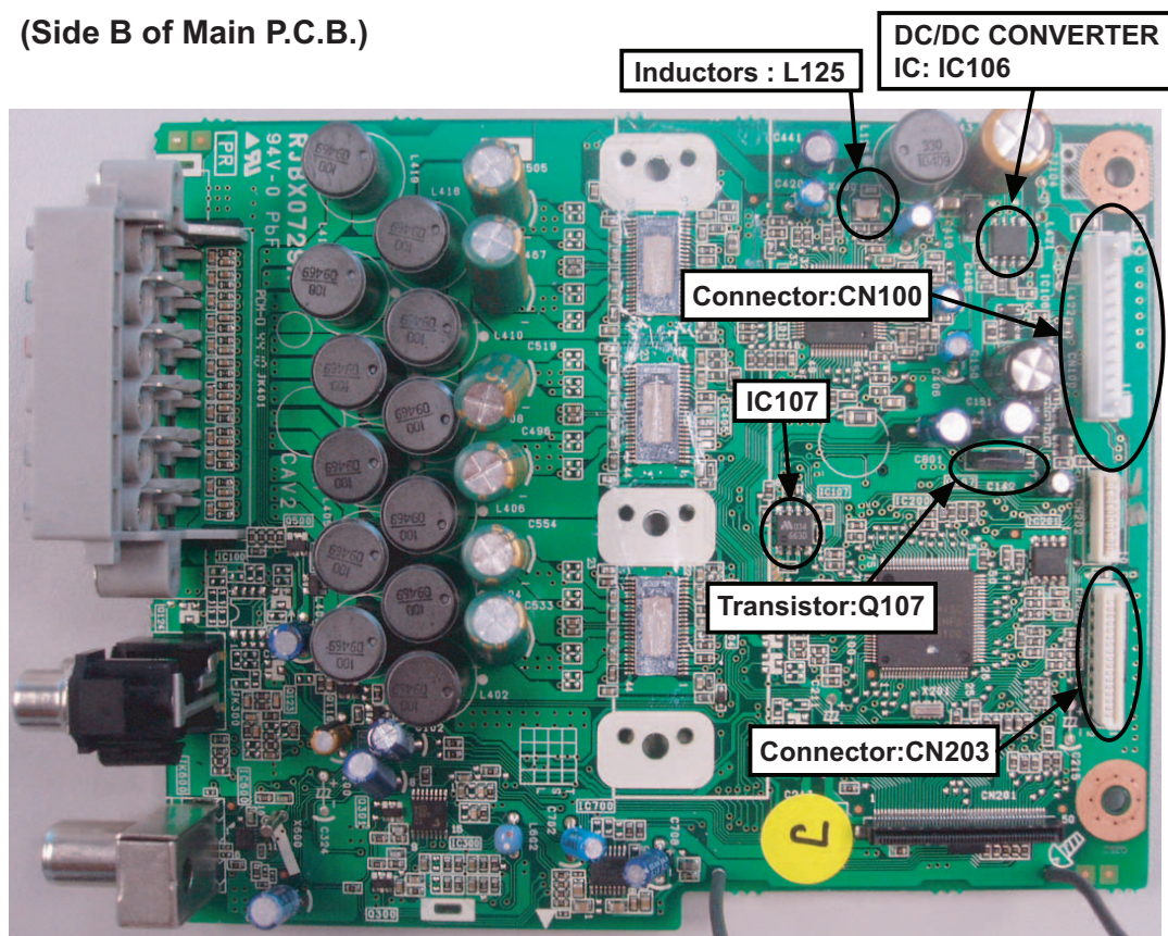
Fig. 2. Main P.C.B.
