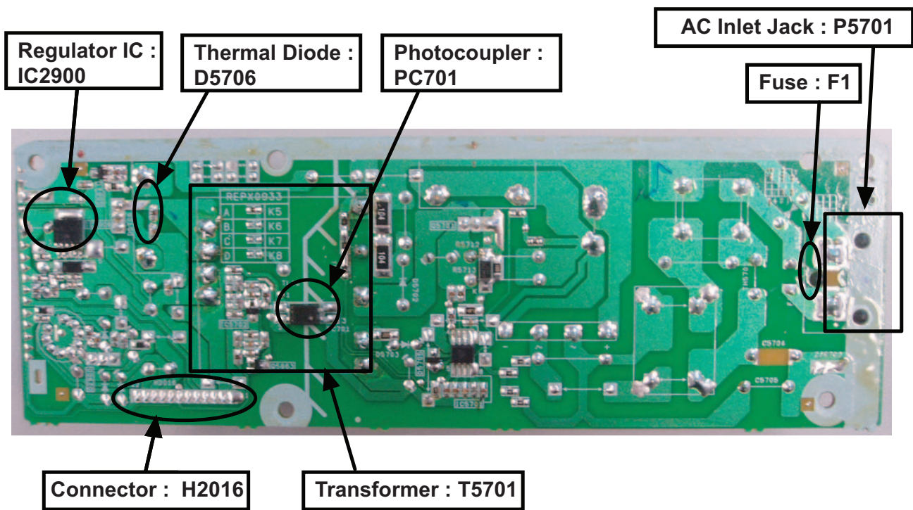
Fig. 1. SMPS P.C.B.
