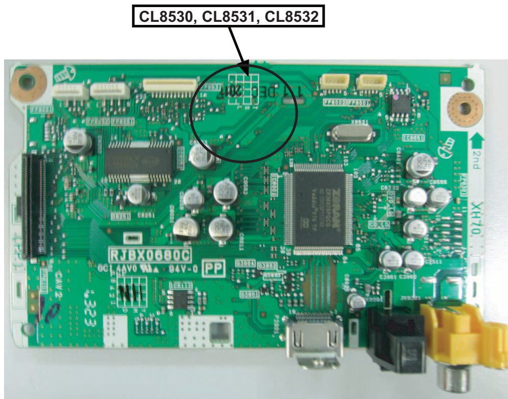
Fig. 3. Backend P.C.B.
