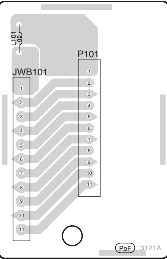
D TUNER EXTENT P.C.B (REP4027C-S)
