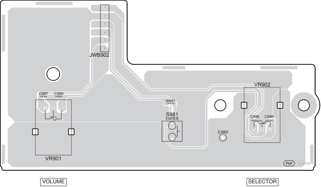
H VOLUME P.C.B (REP4027C-S)
