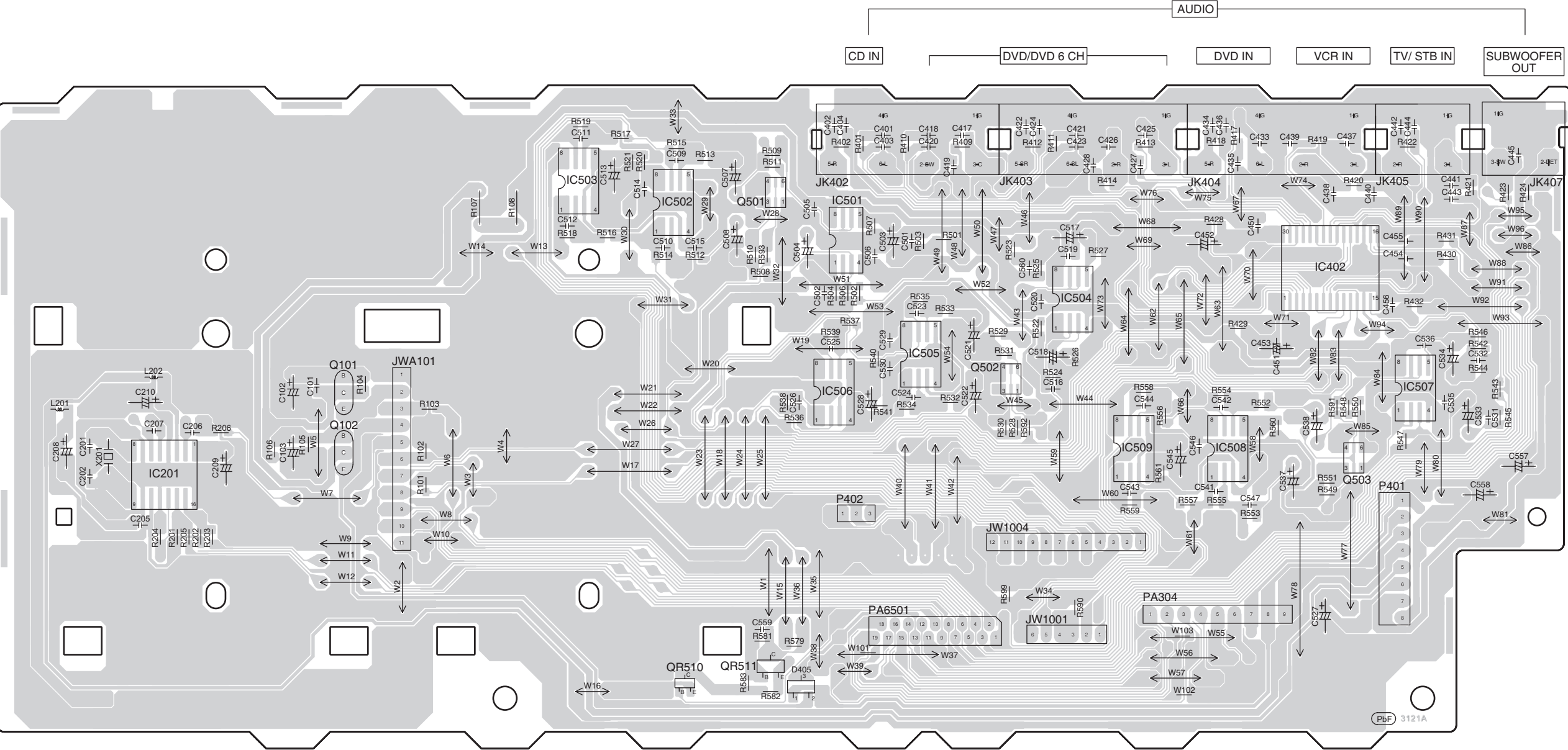
C INPUT P.C.B (REP4027C-S)
