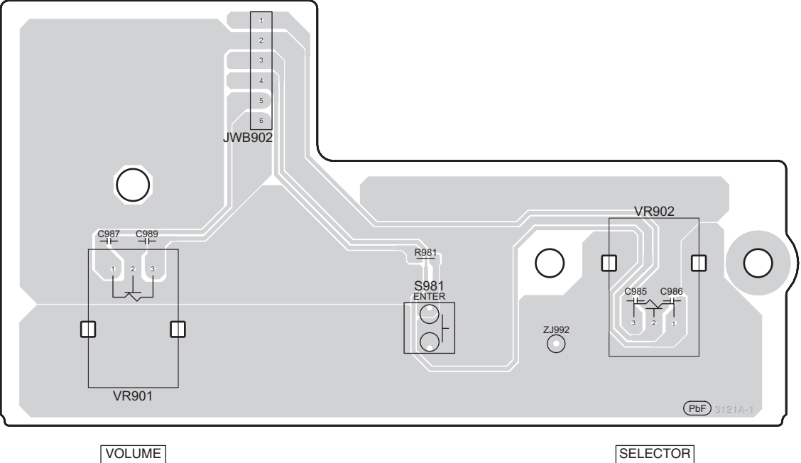
H VOLUME P.C.B (REP4027D-S)
