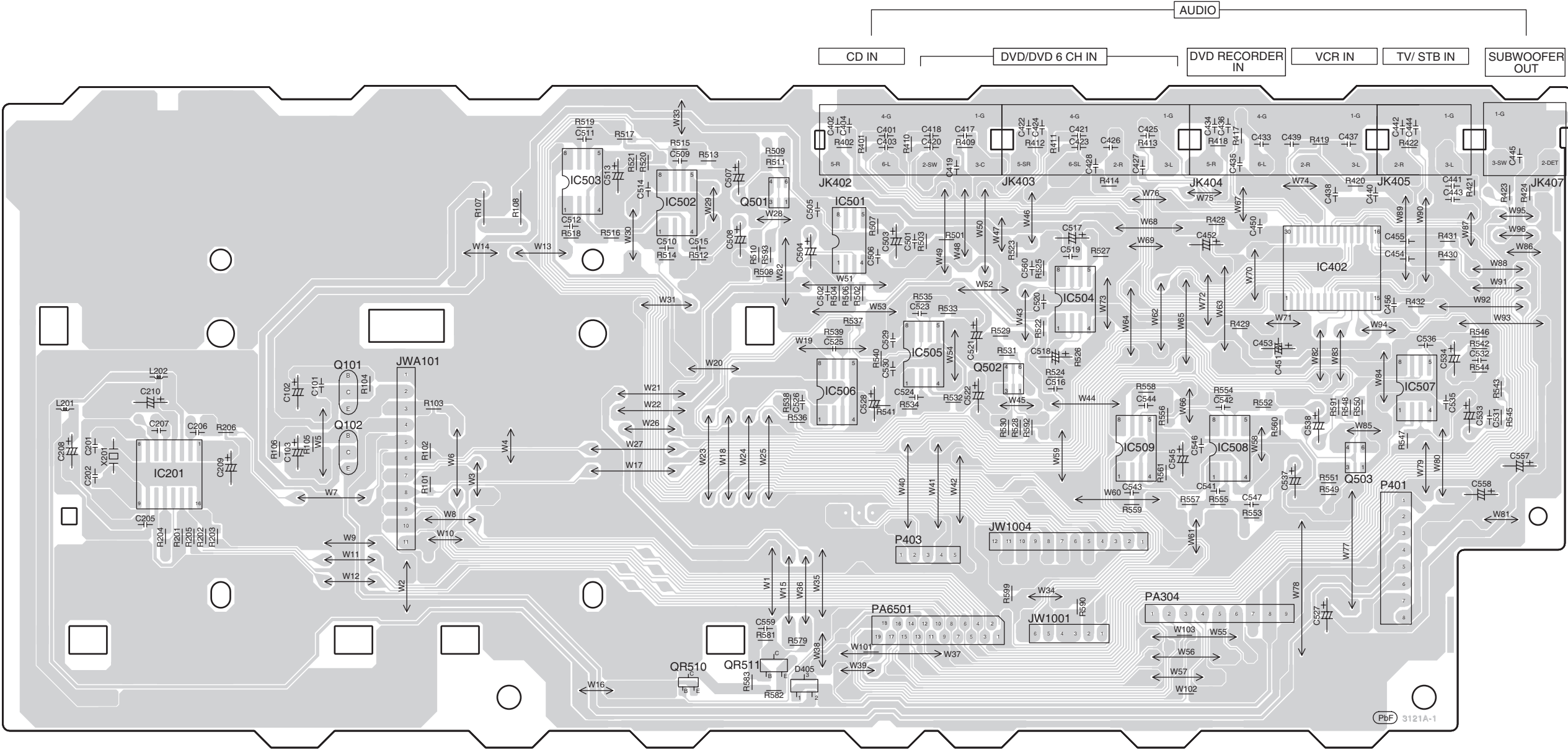
C INPUT P.C.B (REP4027D-S)
