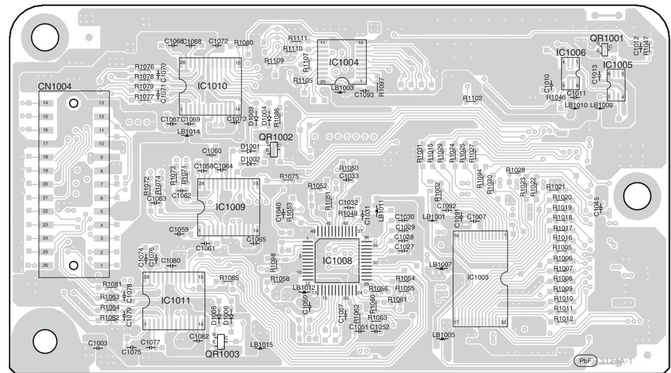
A DSP P.C.B (REP4028A-T)
