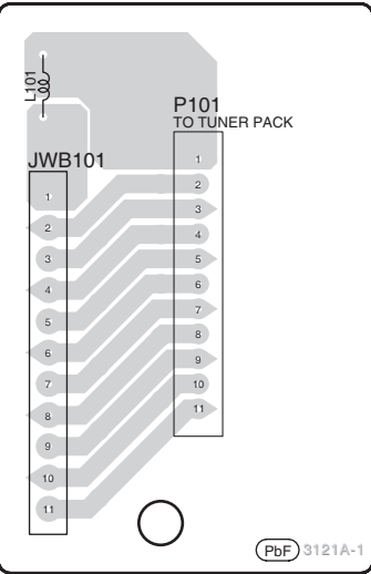
D TUNER EXTENT P.C.B (REP4027D-S)
