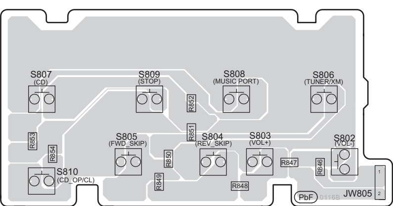
H TACT SWITCH P.C.B (REPV0116B)
