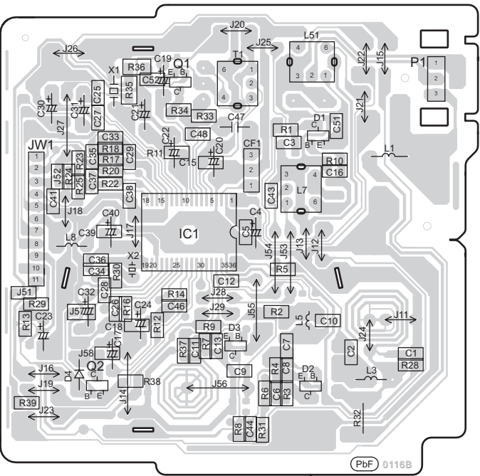
C TUNER P.C.B (REPV0116B)
