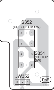
J MOTOR P.C.B (REPV0116B)
