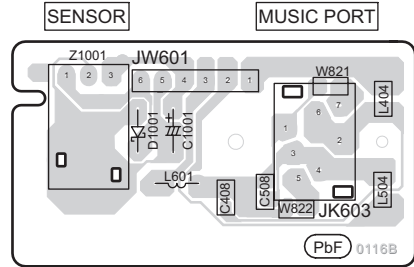
K SENSOR P.C.B (REPV0116B)
