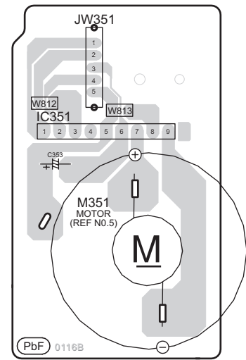
J MOTOR P.C.B (REPV0116B)
