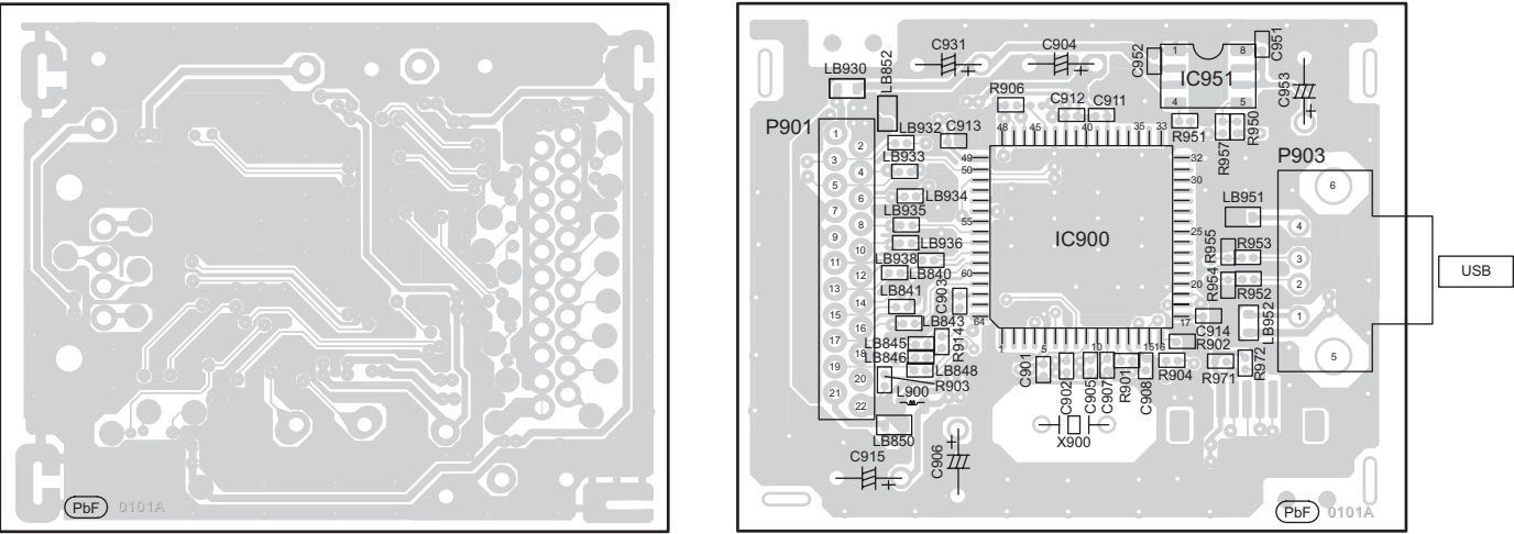
B USB P.C.B (REPV0101A)
