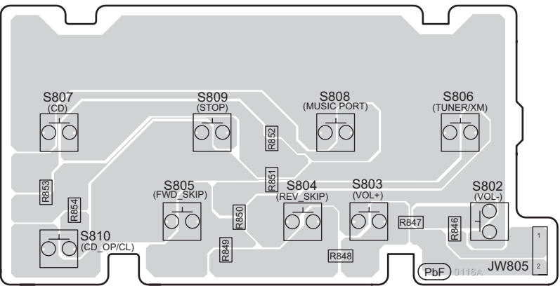
H TACT SWITCH P.C.B (REPV0116A)
