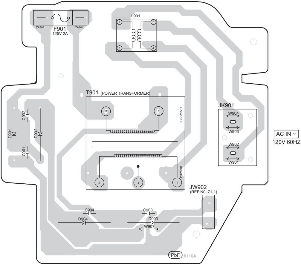
L TRANSFORMER P.C.B (REPV0116A)
