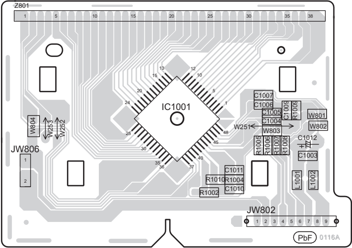
E PANEL P.C.B (REPV0116A)
