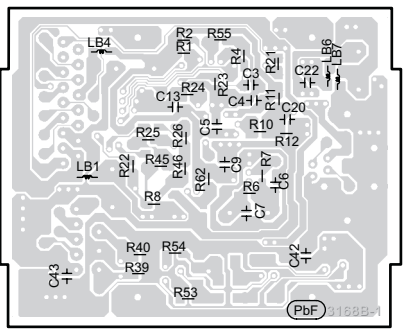
B XM MODULE P.C.B (REP4222B)
