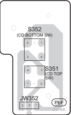
J MOTOR P.C.B (REPV0116A)
