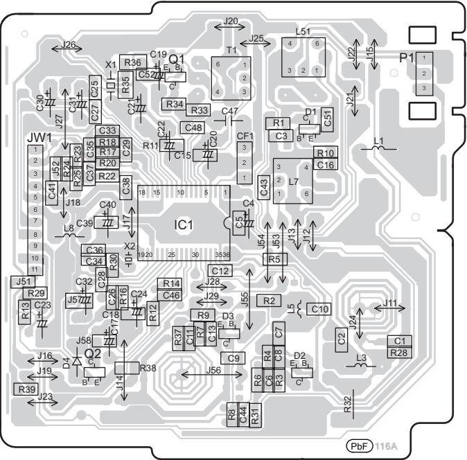
C TUNER P.C.B (REPV0116A)
