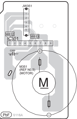
J MOTOR P.C.B (REPV0116A)
