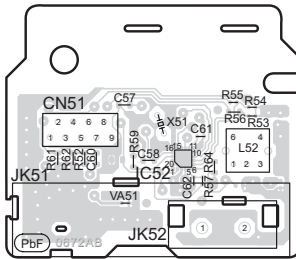
D TUNER P.C.B. (REPX0817HB...EB/EG) (REPX0817LB...EP)
