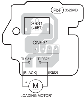
G MOTOR P.C.B. (REP4776AD)
