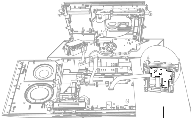
CD Interface P.C.B. (Step 15)
