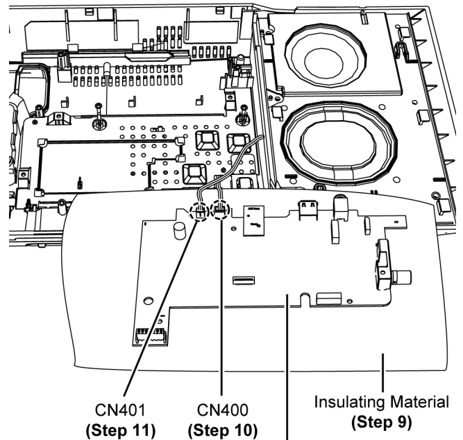
Main P.C.B.
