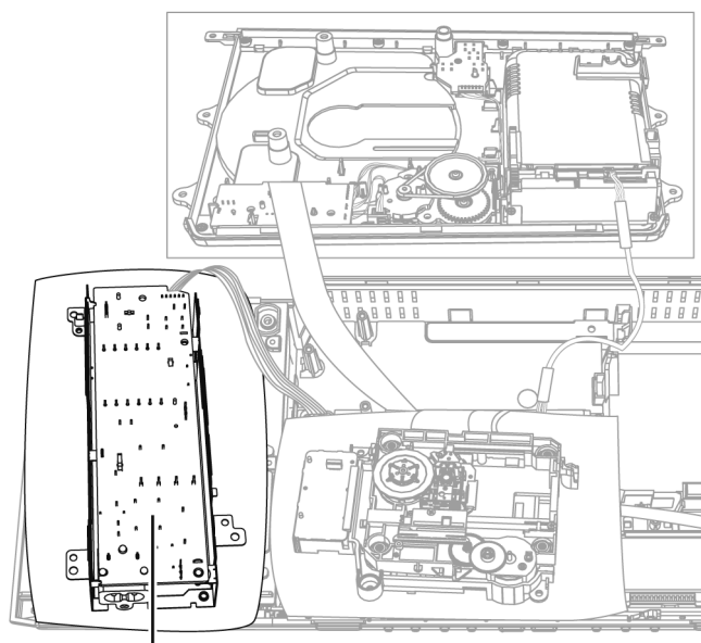
SMPS P.C.B. (Step 20)
