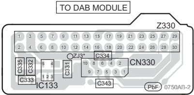
D DAB BRIDGE P.C.B. (REPX0914BB)
