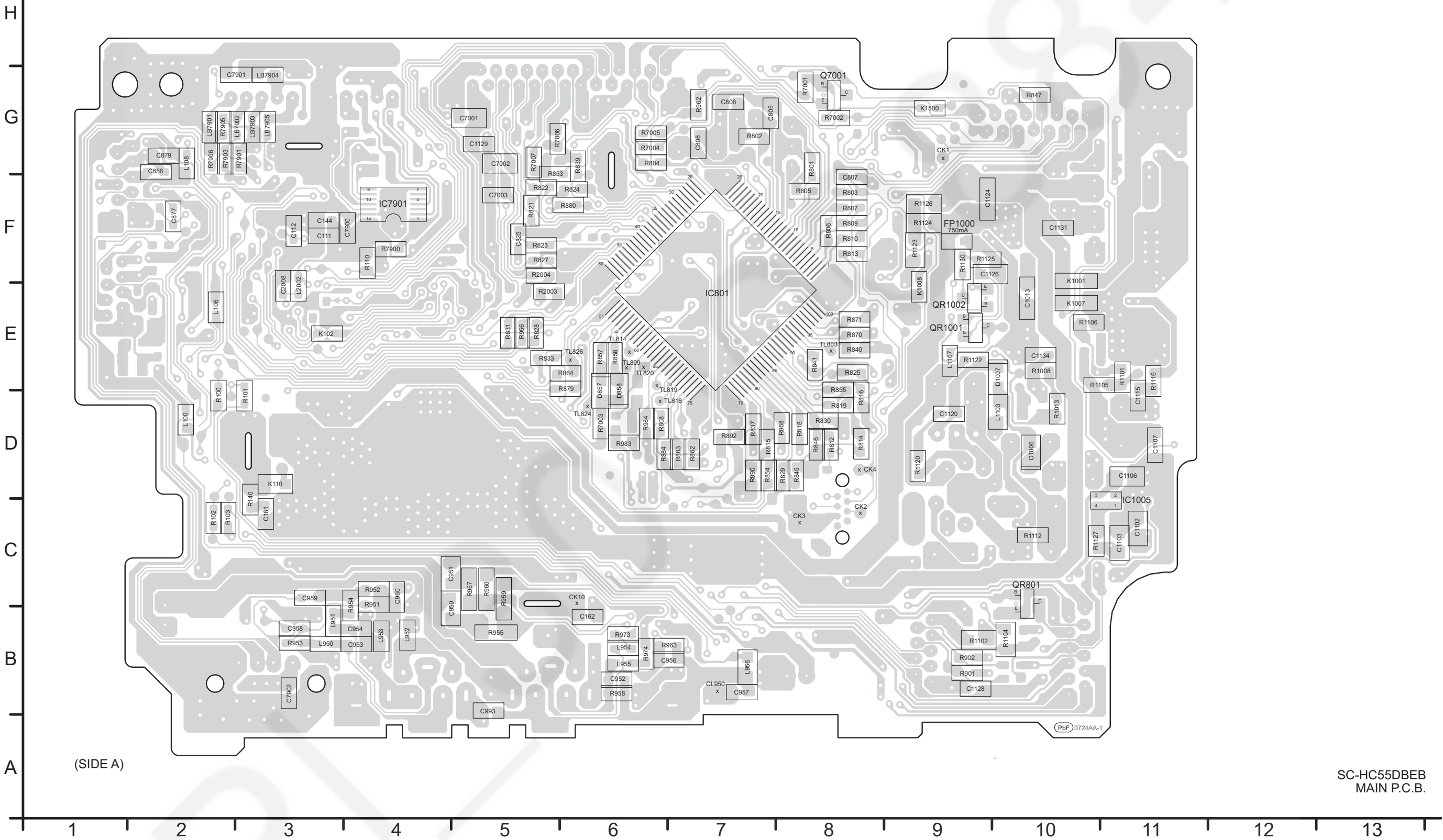
B MAIN P.C.B. (REPX0915MA)
