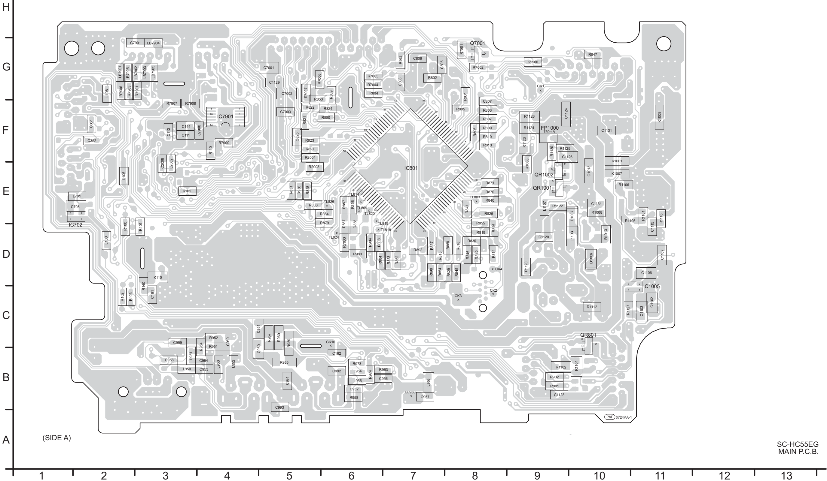
B MAIN P.C.B. (REPX0915LA)
