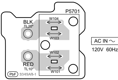
K AC INLET P.C.B. (REP4527B-P)
