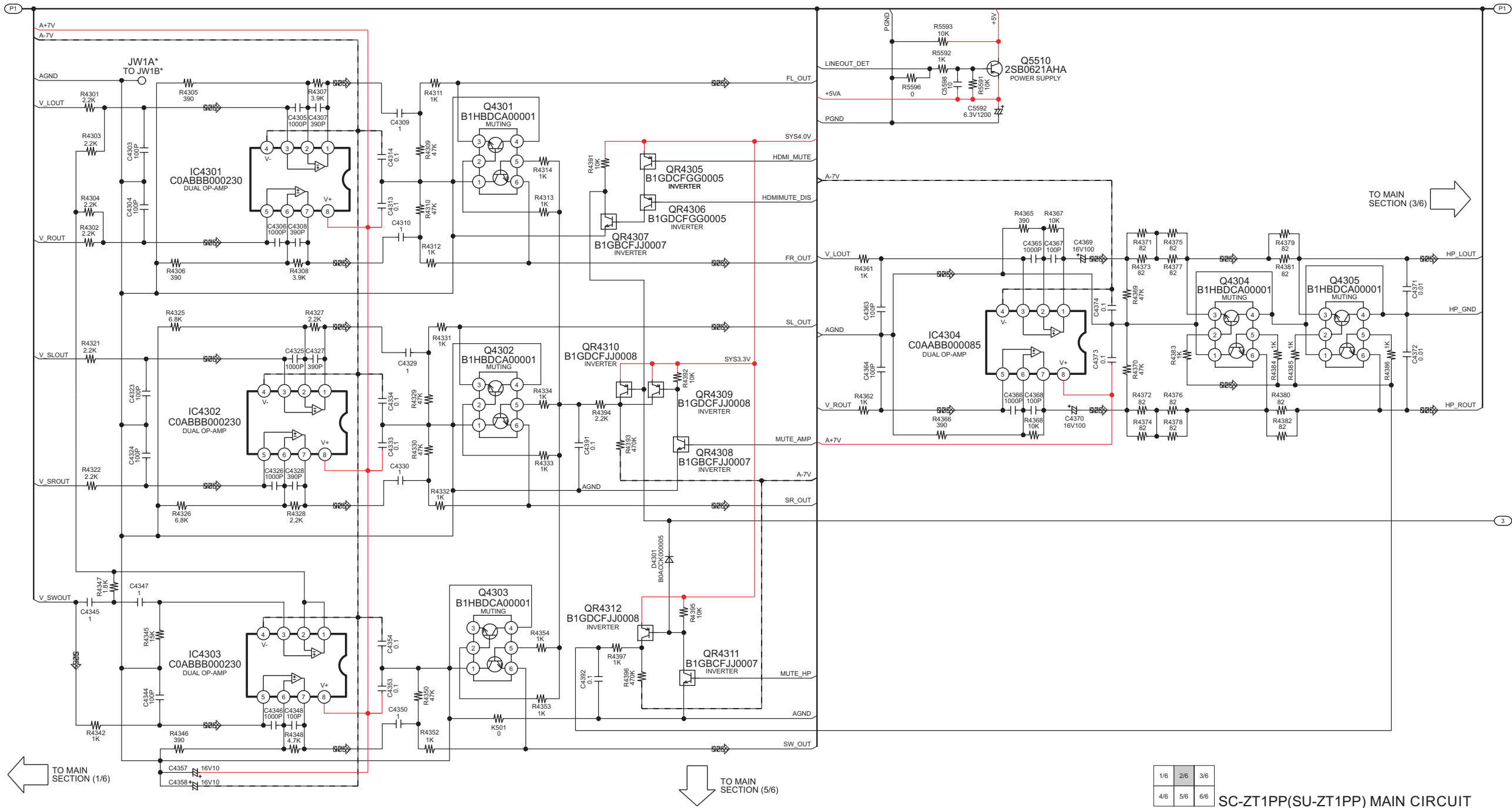
SC-ZT1PP(SU-ZT1PP) MAIN CIRCUIT
