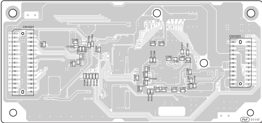
B DSP P.C.B. (REPV0114F-T)
