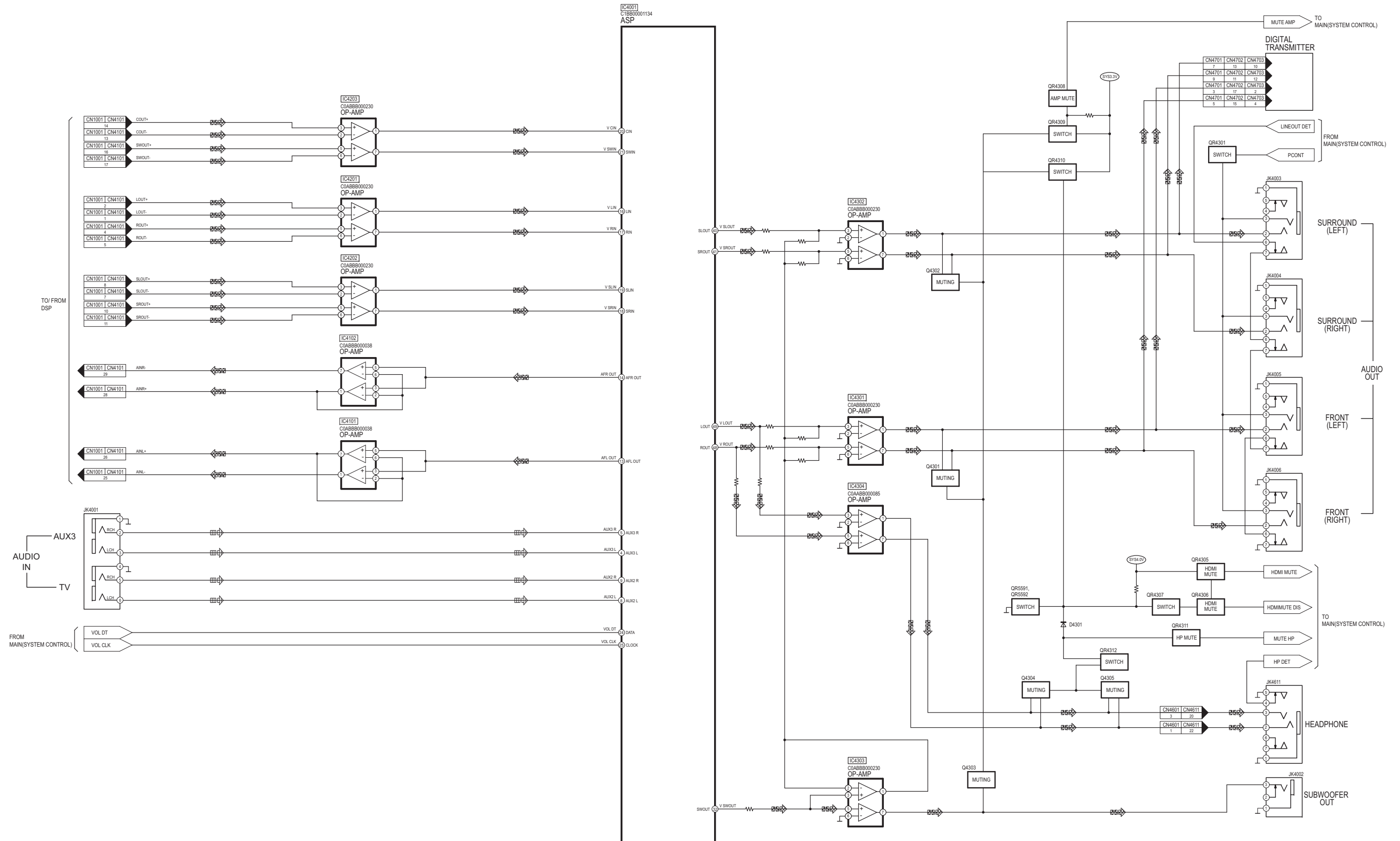
SC-ZT2PP(SU-ZT2PP) MAIN(AUDIO) BLOCK DIAGRAM
