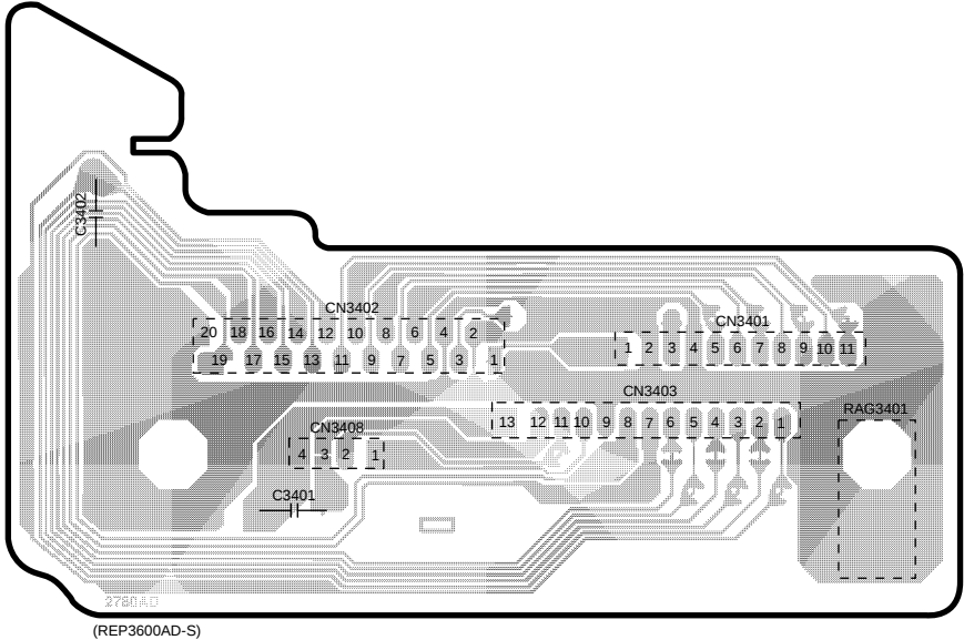
N CONNECTION P.C.B.
