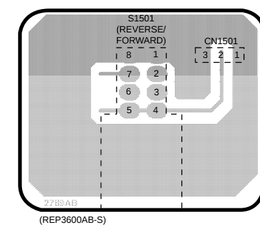
J REVERSE SW P.C.B.
