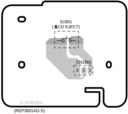
M EJECT SW P.C.B.
