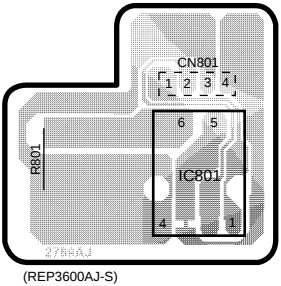
O SENSOR P.C.B.
