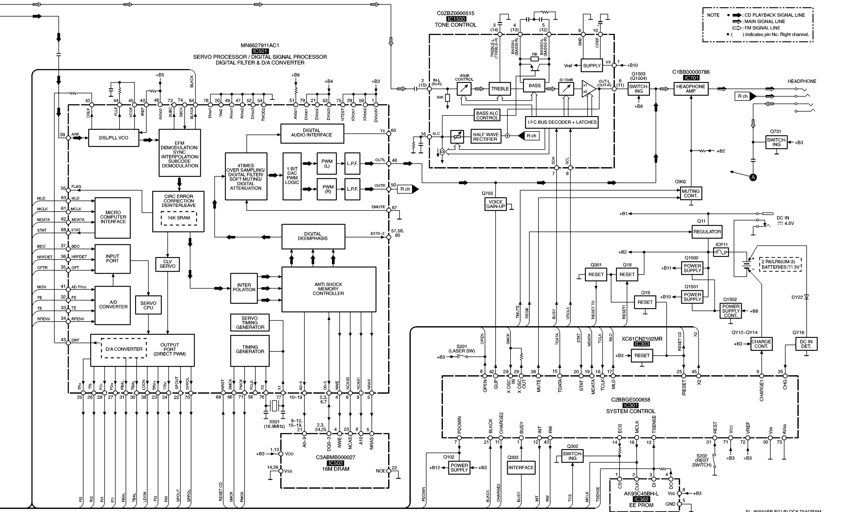
SL-J600V(EB,EG) BLOCK DIAGRAM
