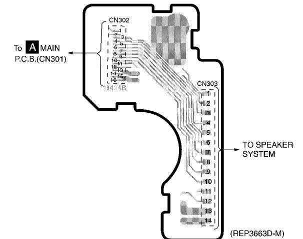
B CONNECTOR P.C.B.(SIDE:A)
