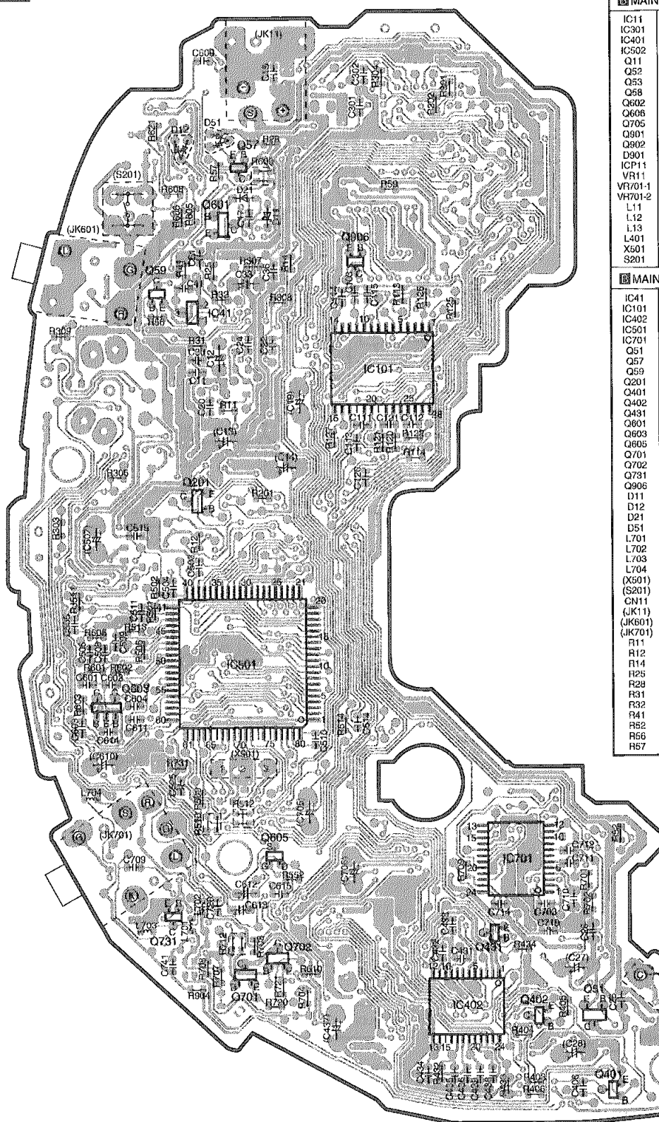
B MAIN P.C.B. (SIDE : B)
