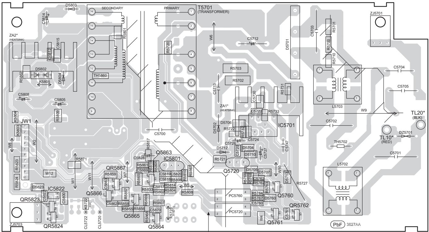
D SMPS P.C.B. (REP4860N)
