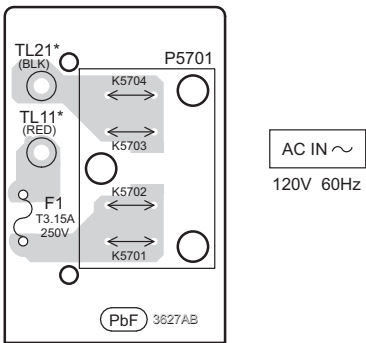
E AC INLET P.C.B. (REP4860N)
