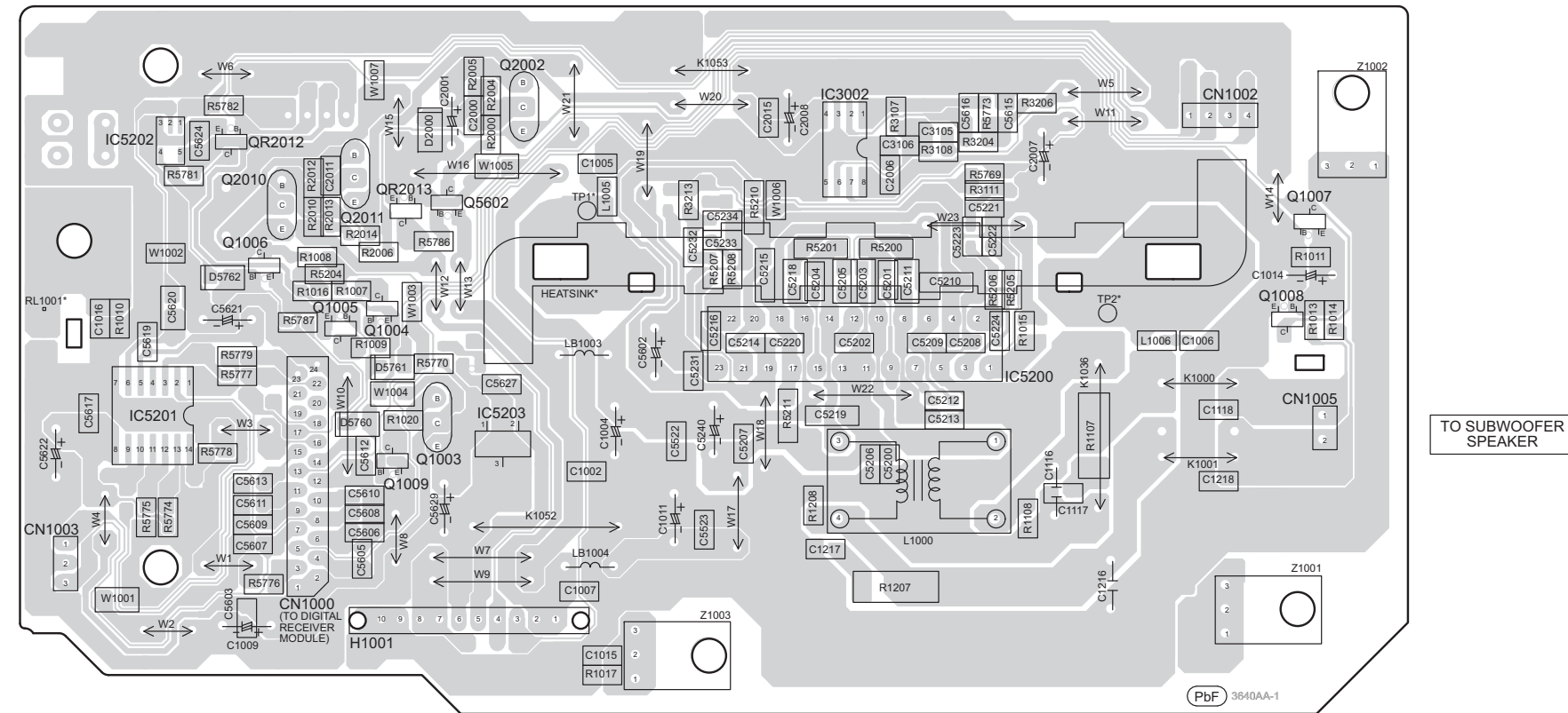
F SW DAMP P.C.B. (REP4869AA)
