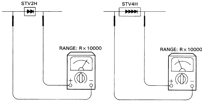
Fig. 74 Checking varistor (1)
