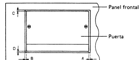
Fig. 11-3 Ajuste de la posición de la puerta
