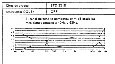
Fig. 11-8 Zona permissible de la respuesta en frecuencia de reproducción
