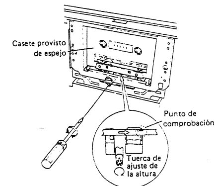
Fig. 11-5 Ajuste del transporte de la cinta
