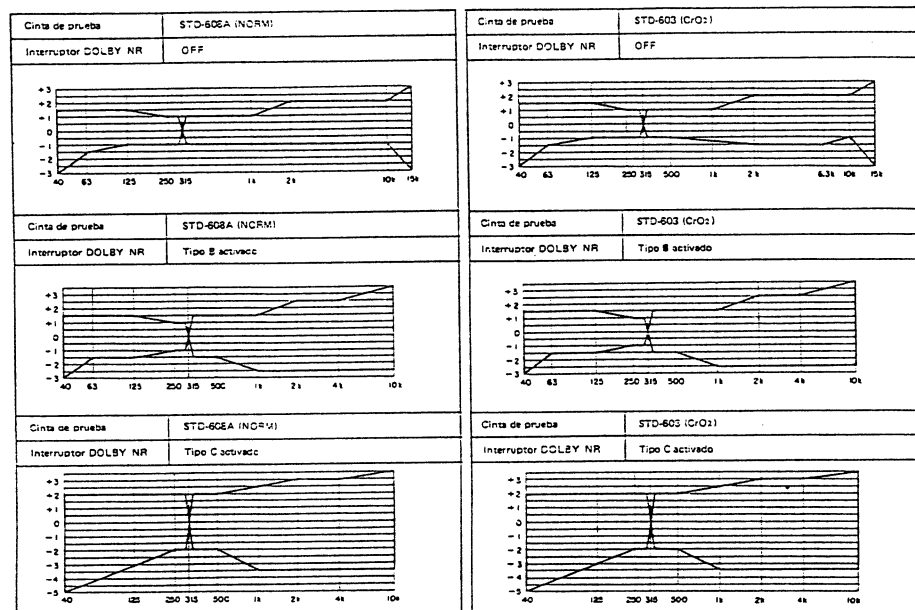
Fig. 11-11 Zona permisible de respuesta en frecuencia de grabación y reproducción (CrO2)
