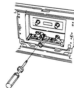
Fig. 11-6 Ajuste del acimut de la cabeza
