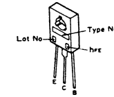
2SD1189
