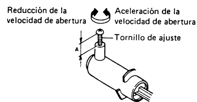
Fig. 11-12 Ajuste del amortiguador neumático
