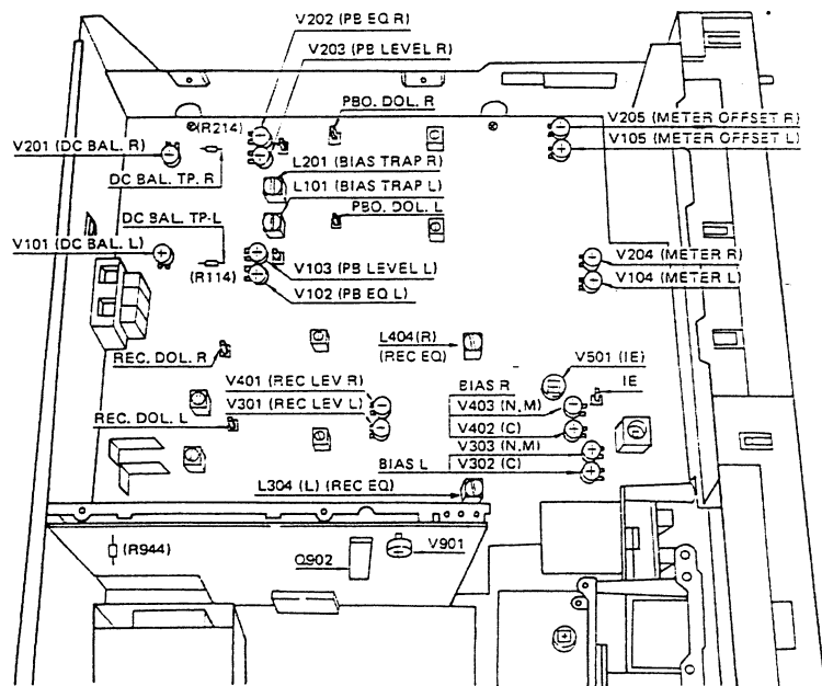
Fig. 11-9 Lugares de ajuste
