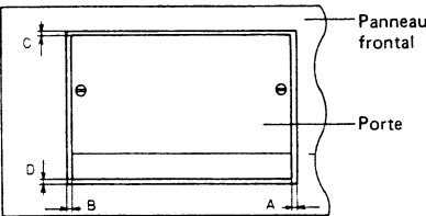
Fig. 11-3 Réglage de la position de la porte
