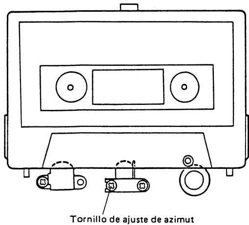
Figura 9-4 Ajuste de azimuth de la cabeza
