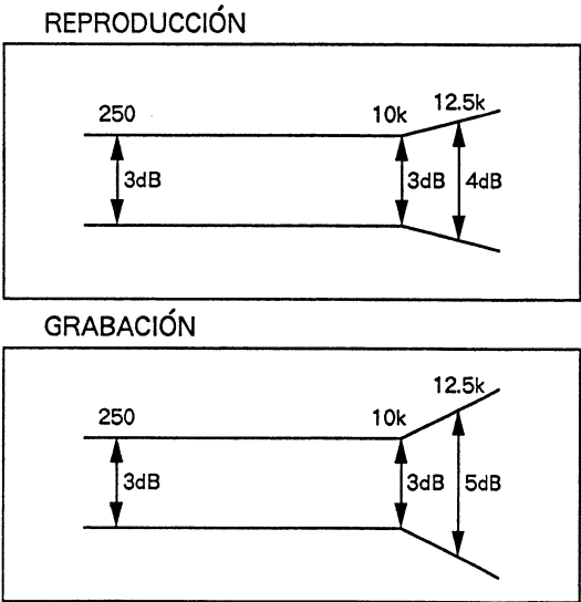
Figura 9-5 Zona permisible de respuesta de frecuencia de reproducción
