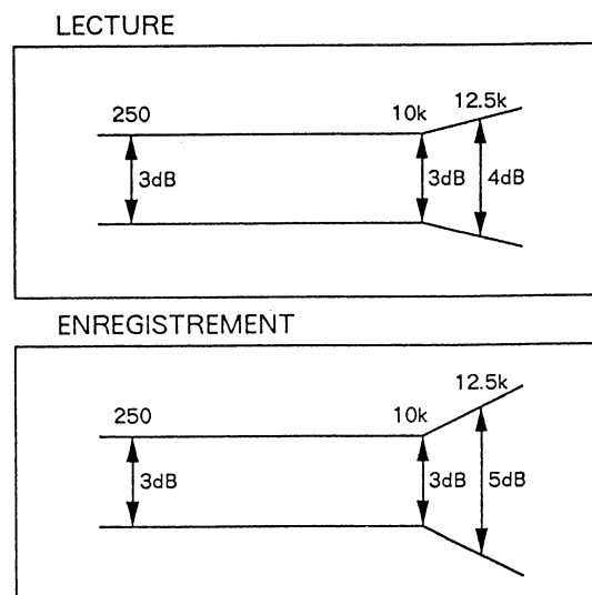
Fig. 7-4 Zone de réponse en fréquence
