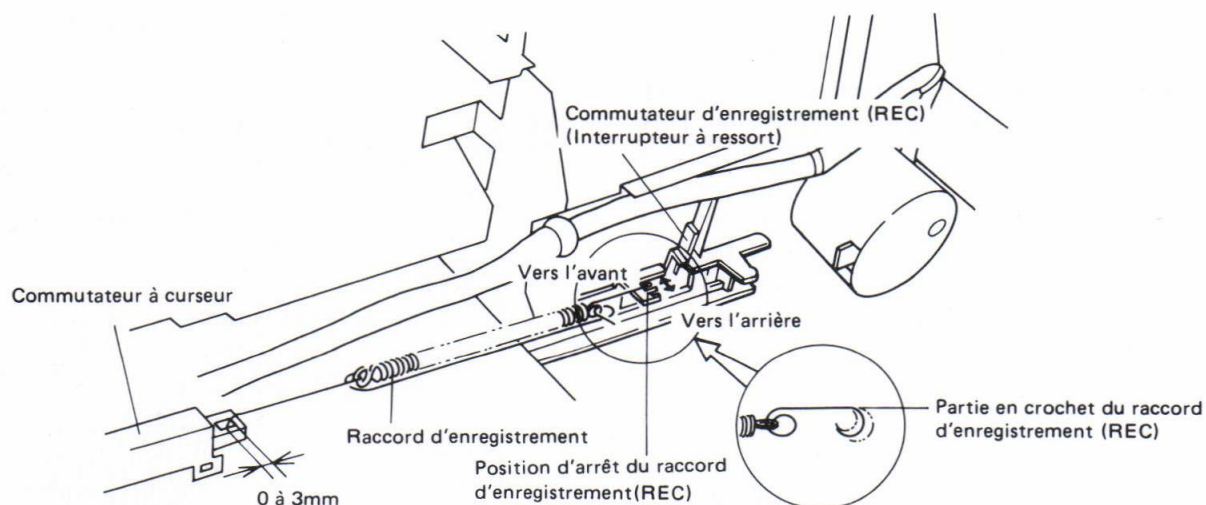
Fig. 11-4 Contrôle et réglage du raccord d'enregistrement
