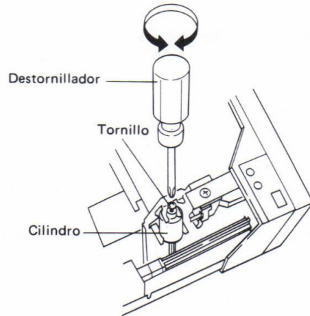
Fig. 11-3 Comprobación y ajuste del amortiguamiento de la puerta
