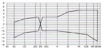
Fig. 11-10 Zone de réponse en fréquence admissible de lecture et d'enregistrement (CrO 2 )
