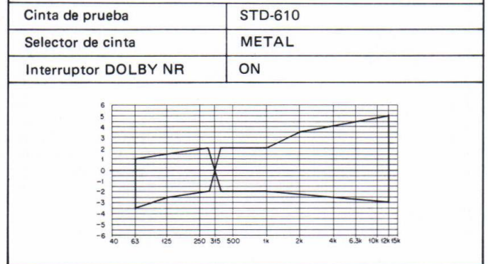
Fig. 11-11 Zona de respuesta de frecuencia de grabación y reproducción permisible (METAL)
