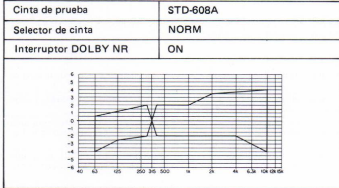
Fig. 11-9 Zona de respuesta de frecuencia de grabación y reproducción permisible (NORM)
