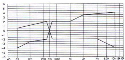
Fig. 11-9 Zone de réponse en fréquence admissible de lecture et d'enregistrement (NORM)
