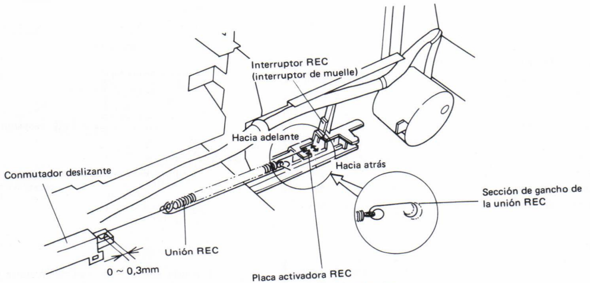
Fig. 11-4 Comprobación y ajuste de la union de grabacion
