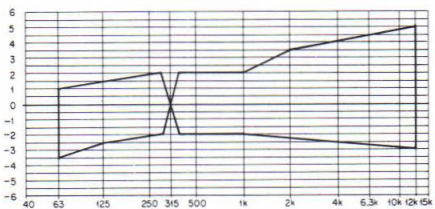
Fig. 11-11 Zone de réponse en fréquence admissible de lecture et d'enregistrement (METAL)
