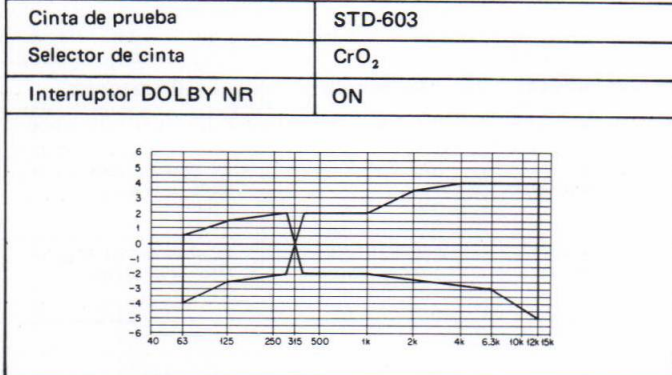
Fig. 11-10 Zona de respuesta de frecuencia de grabación y reproducción permisible (CrO 2 )
