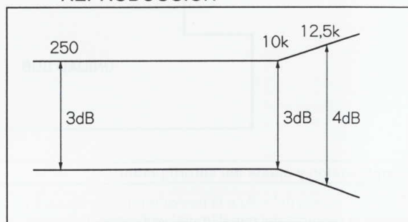
Fig. 4 Cintas de prueba STD-331E
