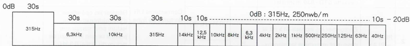
Fig. 4 Cassette d'essai STD-331E
