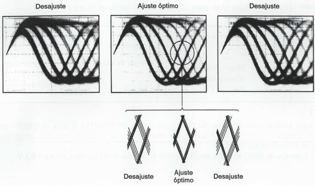
Figura 5 Patron optico
