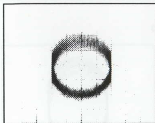
Ganancia óptima
