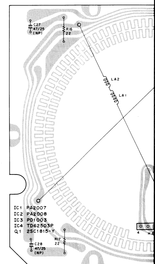
MOTOR (PXM-144)
