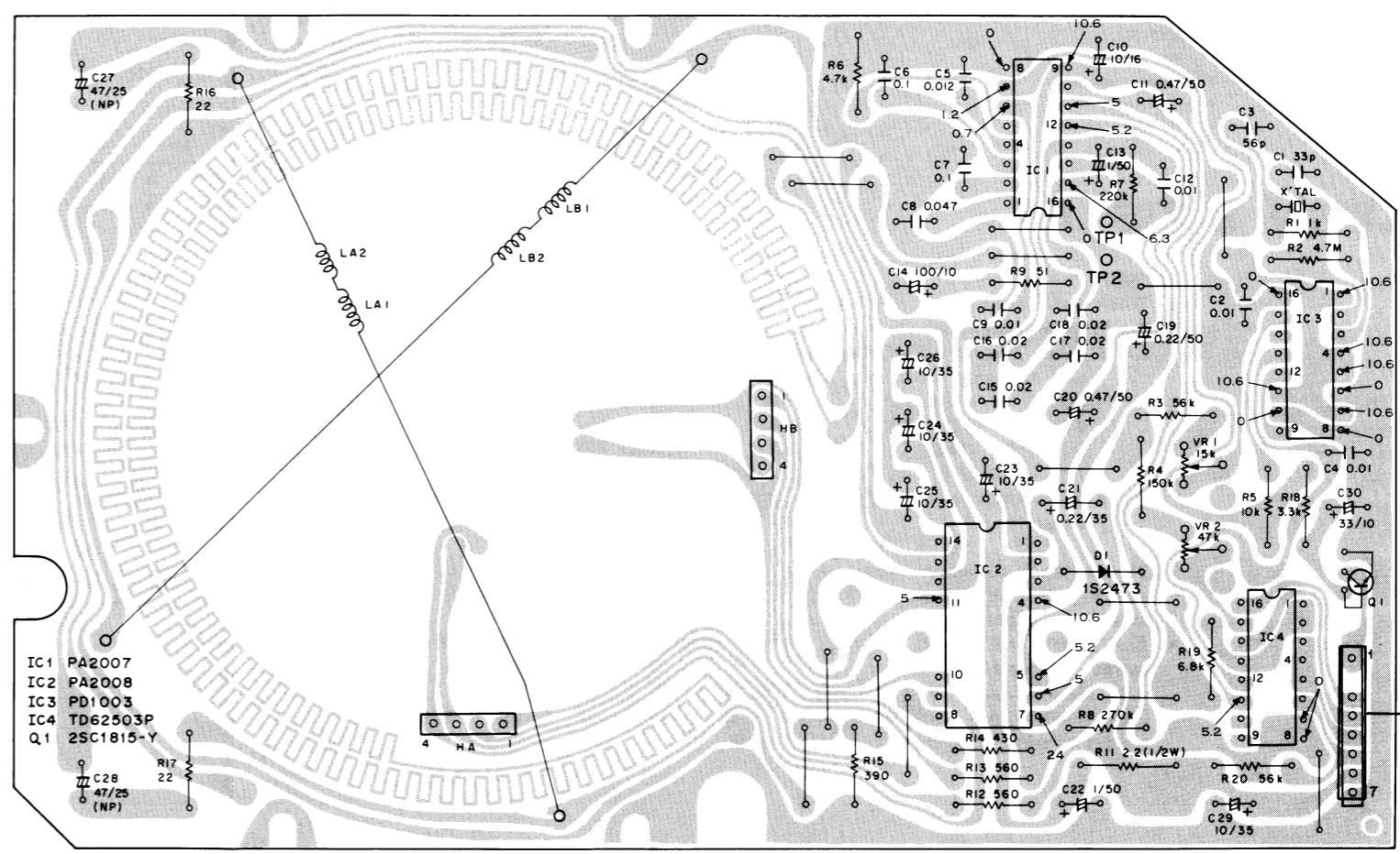
MOTOR (PXM-144)
