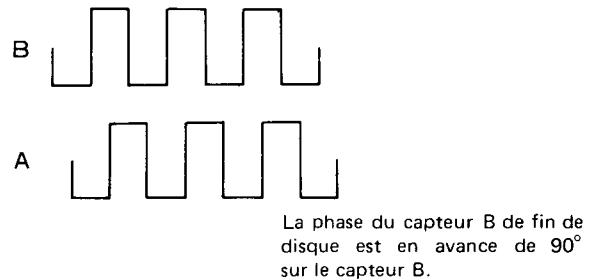
Fig. 14-4 Forme d'onde de sortie 2
