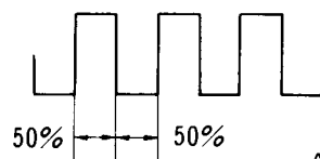
Fig. 14-3 Forma de ondas de salida 1
