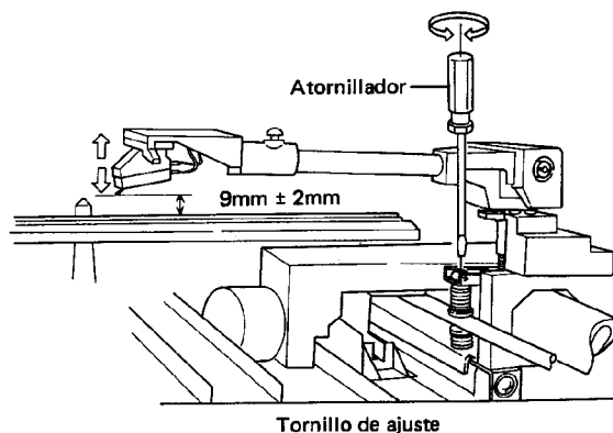
Fig. 11-2 Ajuste de la elevación del brazo
