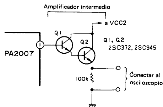
Fig. 11-4 Conectar al amplificador intermedio
