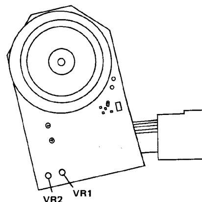
Fig. 11-6 Posiciones de VR1 y VR2
