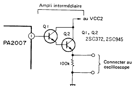
Fig. 11-4 Connexion de l'amplificateur intermédiaire
