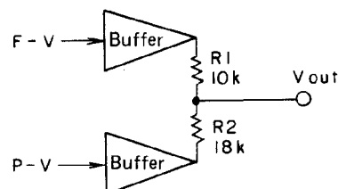
Fig. 4-6 (F-V) + (P-V) circuit
