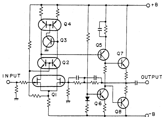
Fig. 5-3 EQ Amplifier
