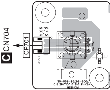
D P.C.B SUB ASSY(VOLUME)
