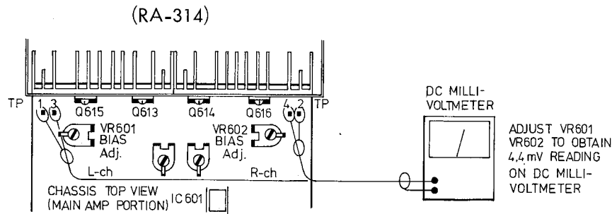
Fig. 1. Power Amplifier Bias Adjustment Hook-up Abb. 1. Messanschluss zur Endverstärker-Vorspannungseinstellung Fig. 1. Réglage de la Polarisation d'Amplificateur de Puissance
