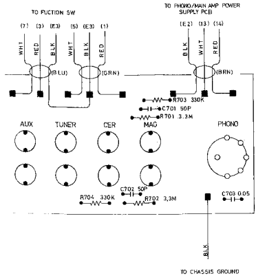
Volume Control Circuit Board Diagram Schaltbild des Lautstärkerger Diagramme de Plaque du Circuit des Réglage de Puissance
