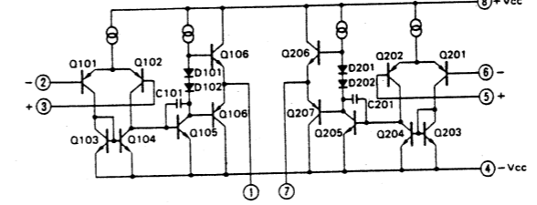
•M5218L(PRE AMP)
