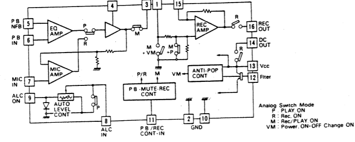
•BA5101(PRE AMP)
