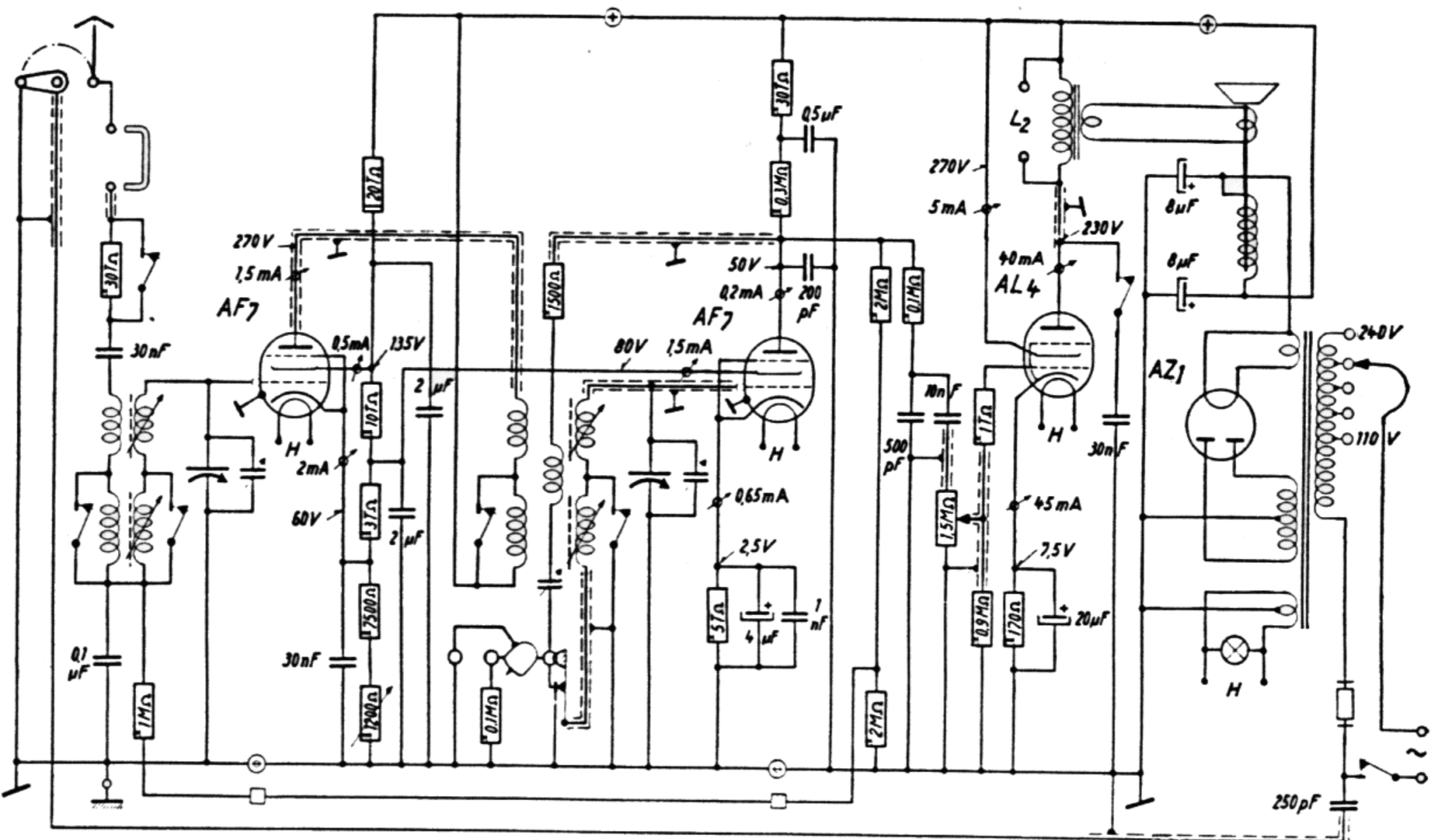
Siemens, Standard 73W, Wechselstrom, 2 Kreise
