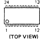
LA9215
