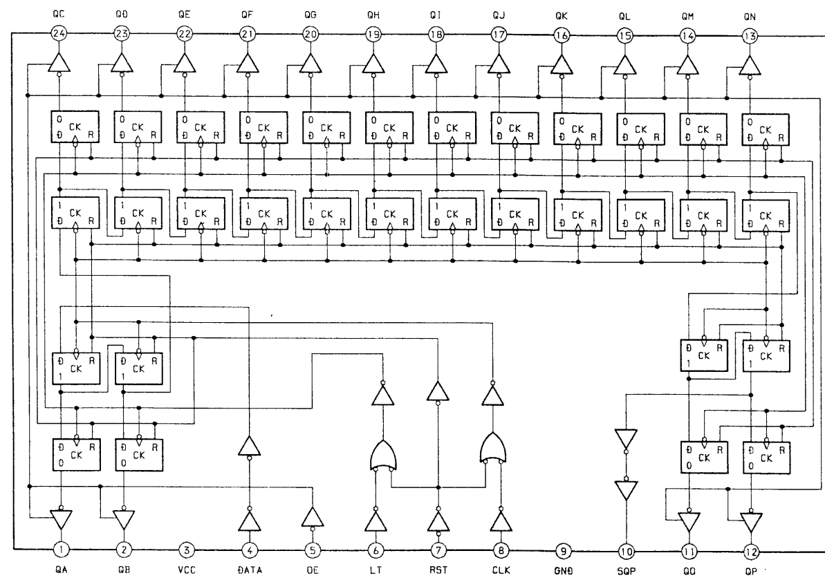
IC702 M66310FP
