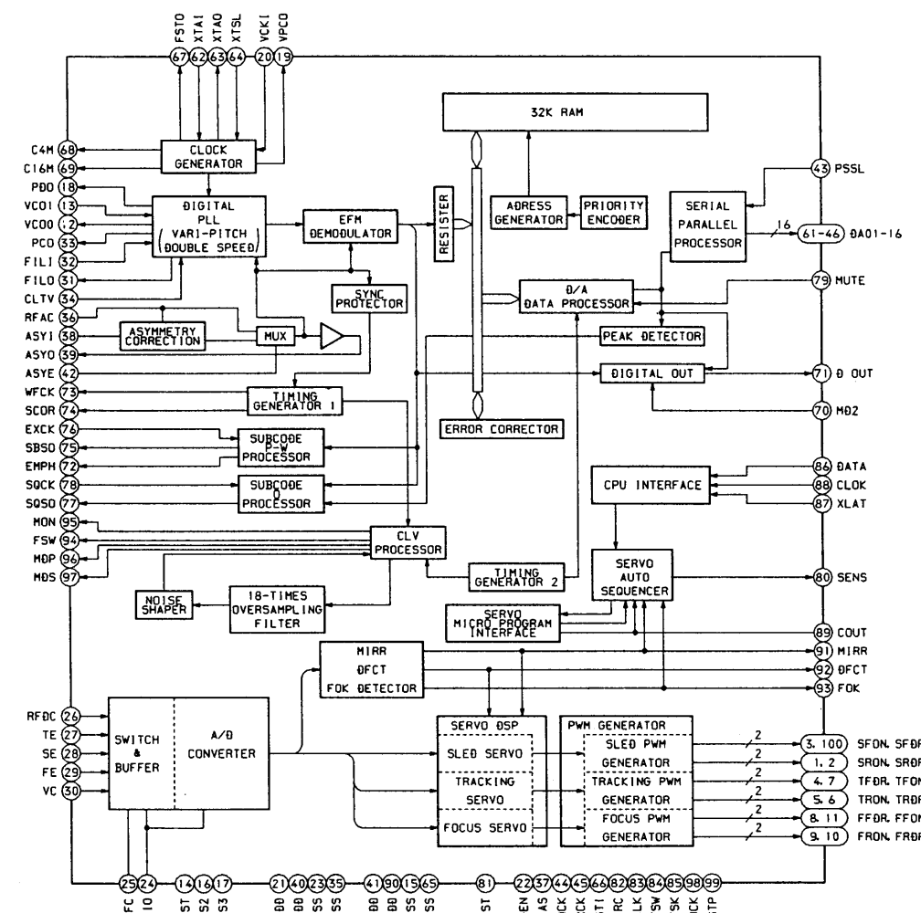
IC101 CXD2545Q
