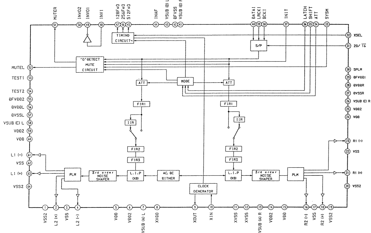
IC613 NJU6355EM-T1
