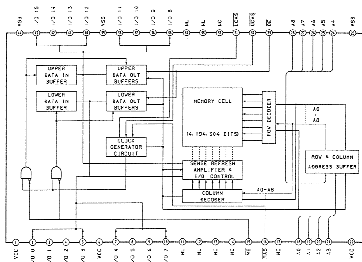
IC601, 603 MSM44260ATP-7L
