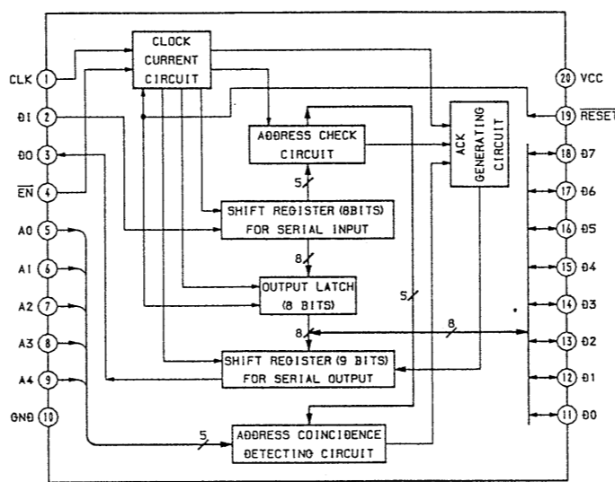
IC903 M66009FP
