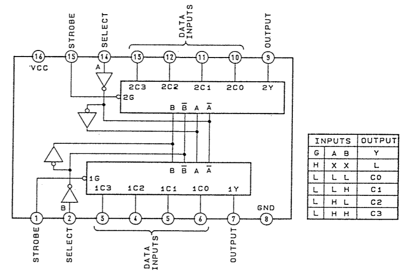
IC906 SN74HC153ANS
