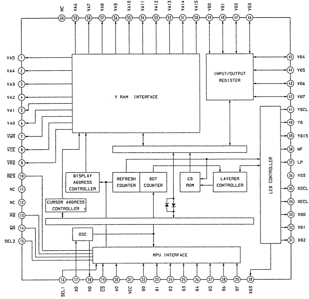
IC610 SED1335F0B
