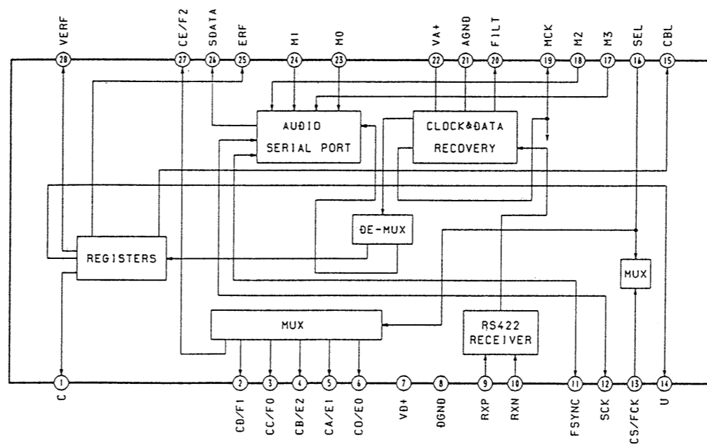
IC901 CS8412-CS
