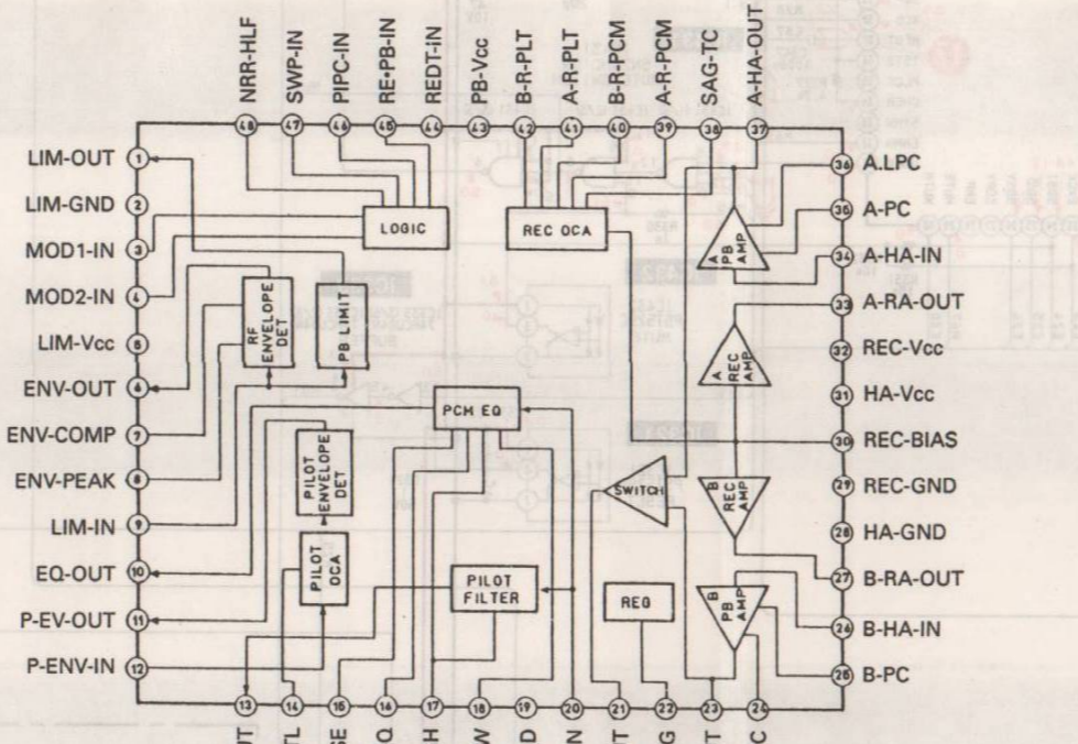
IC1 CXA1364R
