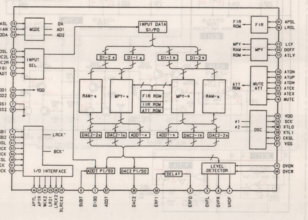
IC306 CXD1136Q
