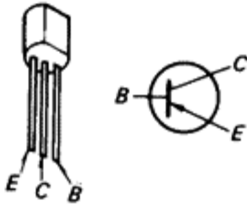
2SA733: Q7
